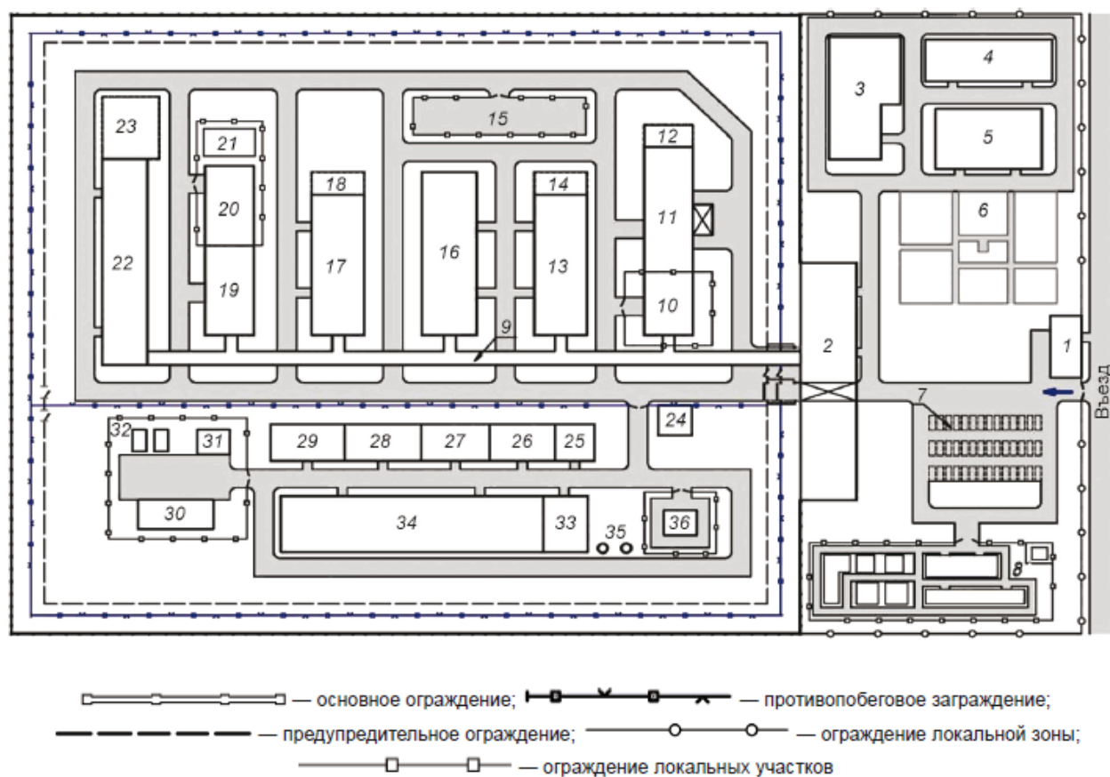
Рисунок Б.1 - Примерная схема планировочной организации земельного участка
