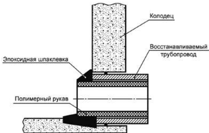
Рисунок 21 - Устройство примыкания с применением эпоксидной шпаклевки - специальные манжеты на основе полиметилметакрилата (рисунок 22);
