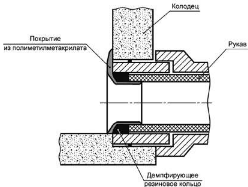
Рисунок 22 - Устройство примыкания с применением манжет на основе полиметилметакрилата - манжеты из нержавеющей стали (рисунок 23).
