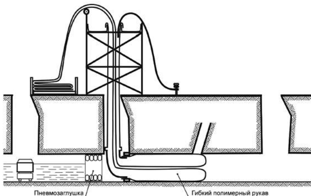
Рисунок 8 - Монтаж гибкого полимерного рукава методом "инверсии"
