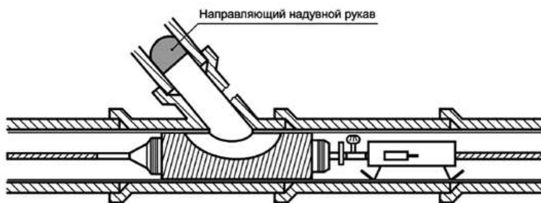
Этап 2. Позиционирование и затвердевание шляпообразной вставки
