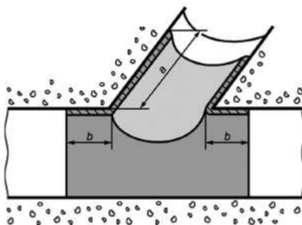
Рисунок 20 - Т-образная манжета
