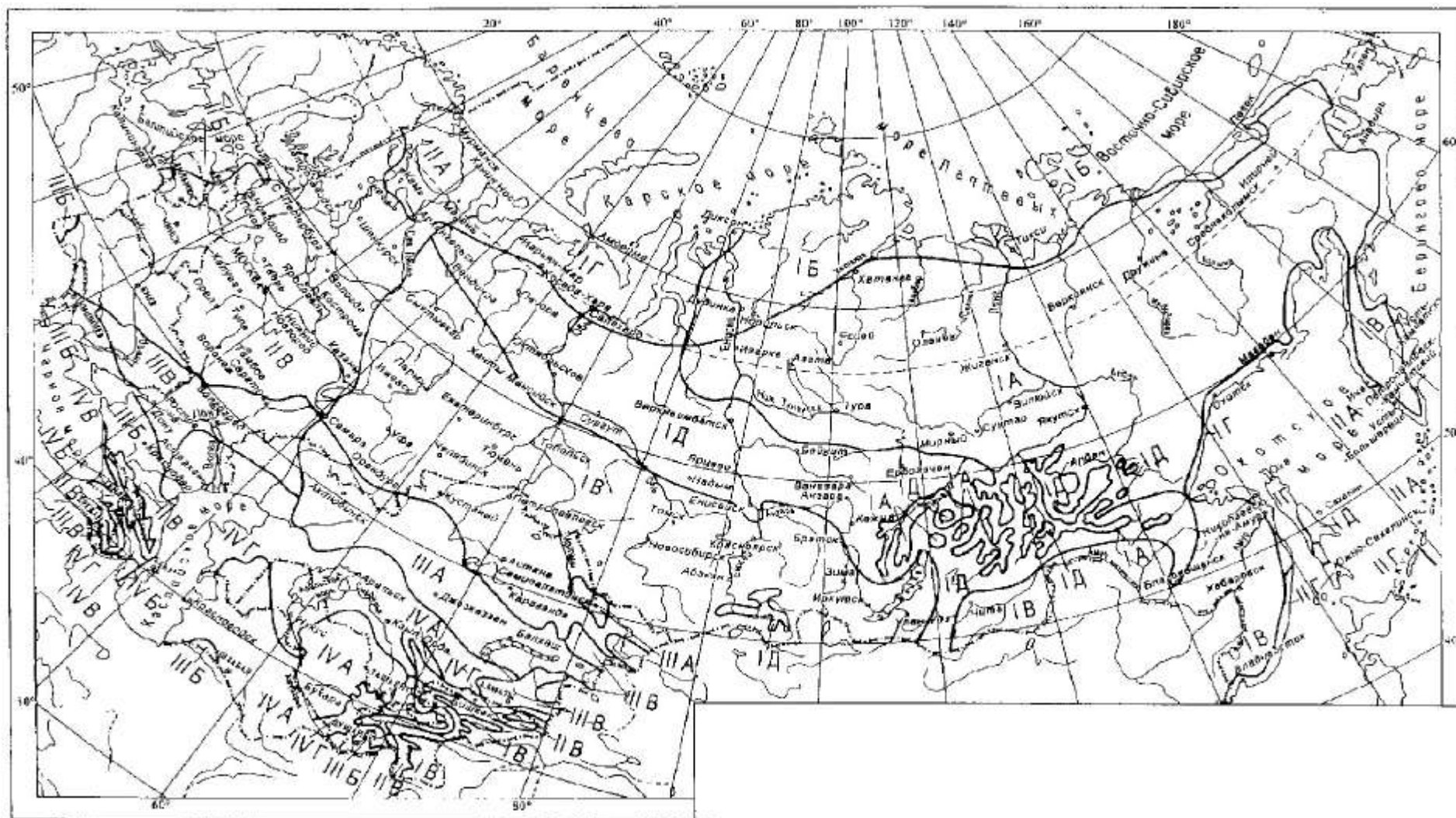
Рисунок А.1 - Схематическая карта климатического районирования территории Российской Федерации для строительства
