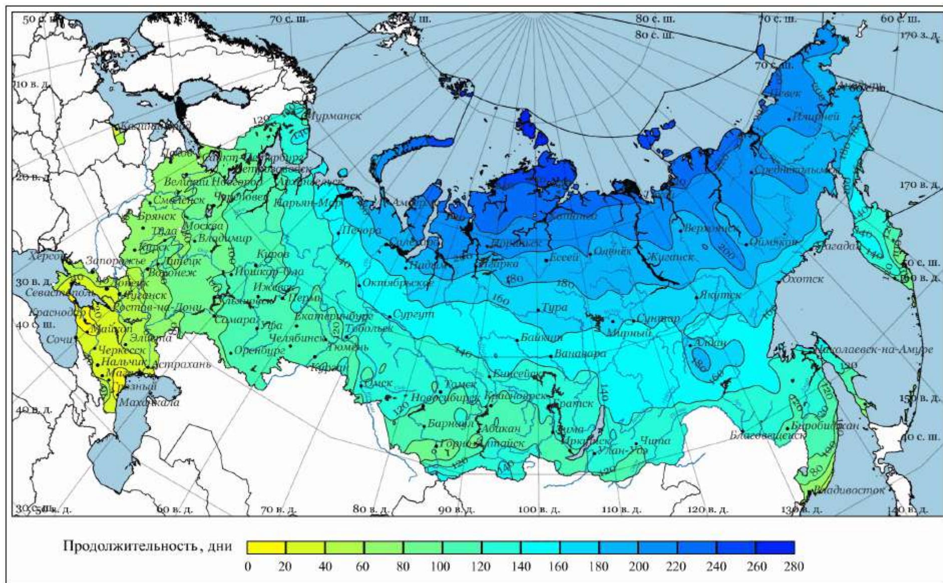
Рисунок А.10 - Схематическая карта районирования по продолжительности периода с устойчивыми морозами, дни Приложение Б
