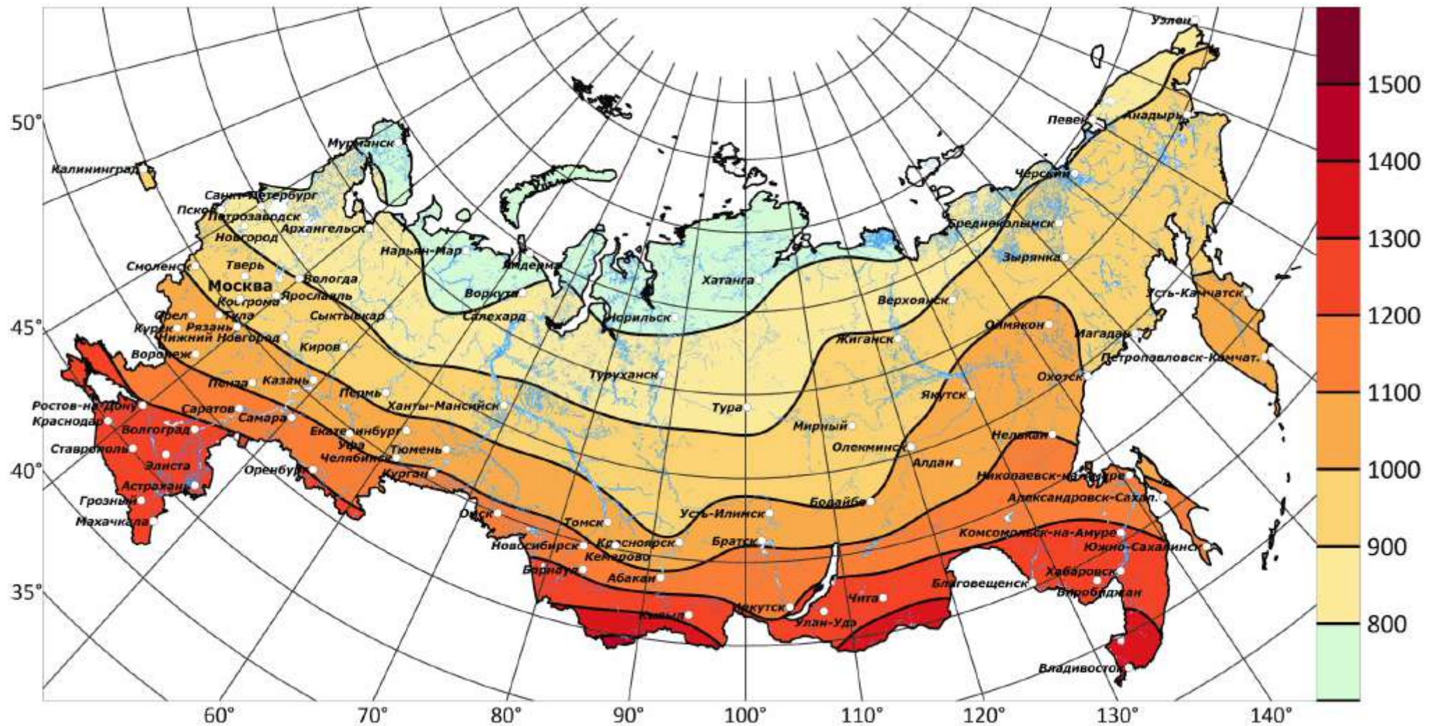
Рисунок А.9 - Схематическая карта районирования по годовому приходу суммарной солнечной радиации, поступающей на горизонтальную
