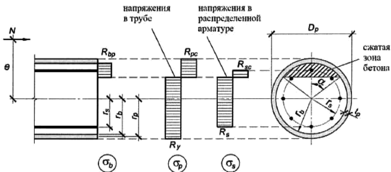
Рисунок 7.3 - Схема усилий и эпюра напряжений в сечении, нормальном к продольной оси внецентренно сжатого трубобетонного элемента, при расчете его по прочности (Измененная редакция, Изм. N 1).
