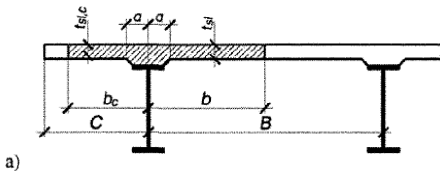
а) - плита с вутами, б) - плита без вутов
