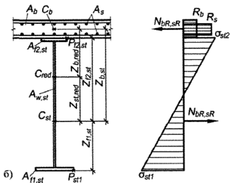
Рисунок 6.13, лист 2
