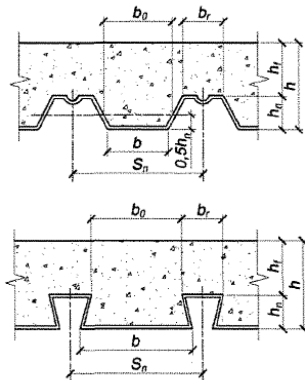
а) - стальной профилированный настил с гофром открытого типа; б) - стальной профилированный настил с гофром закрытого типа
