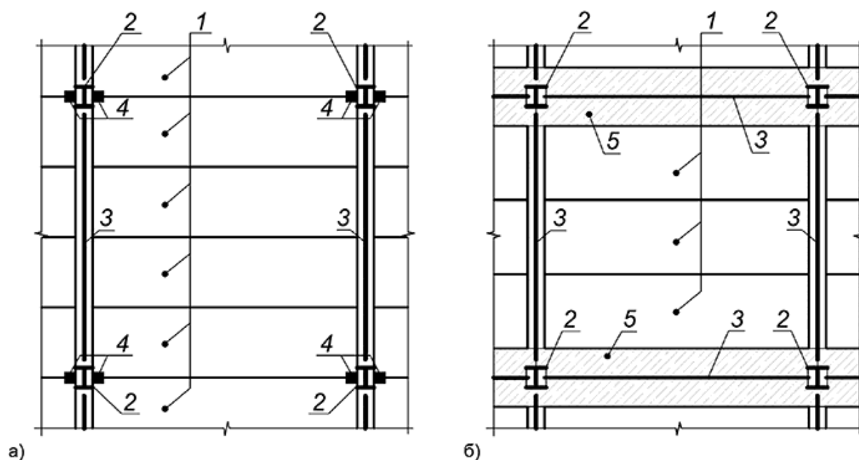
а) фиксация сборных плит путем установки жестких упоров для крайних плит каждого пролета; б) фиксация сборных плит путем создания монолитных участков между крайними плитами и стальными
