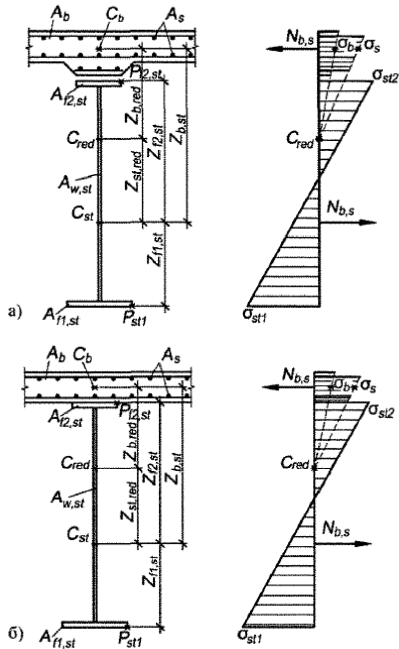
а) - плита с вутами; б) - плита без вутов
