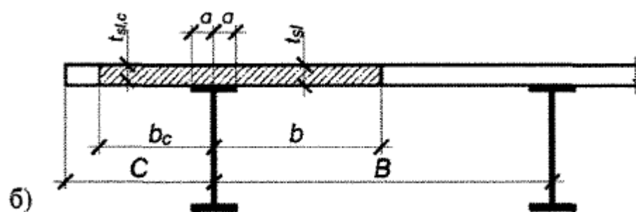
Рисунок 4.5, лист 2
