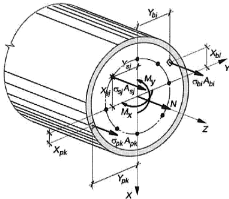
Рисунок 7.4 - Расчетная схема нормального сечения трубобетонного элемента
