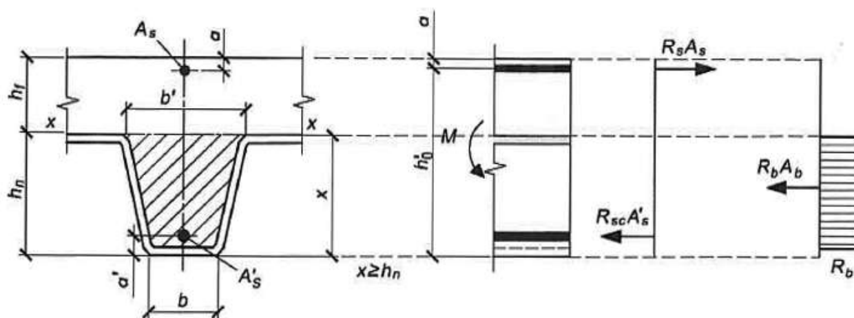
Рисунок 6.7 - Схема усилий в опорном сечении плиты при расположении нейтральной оси на уровне верхней полки профилированного настила (Измененная редакция, Изм. N 1, 2).
