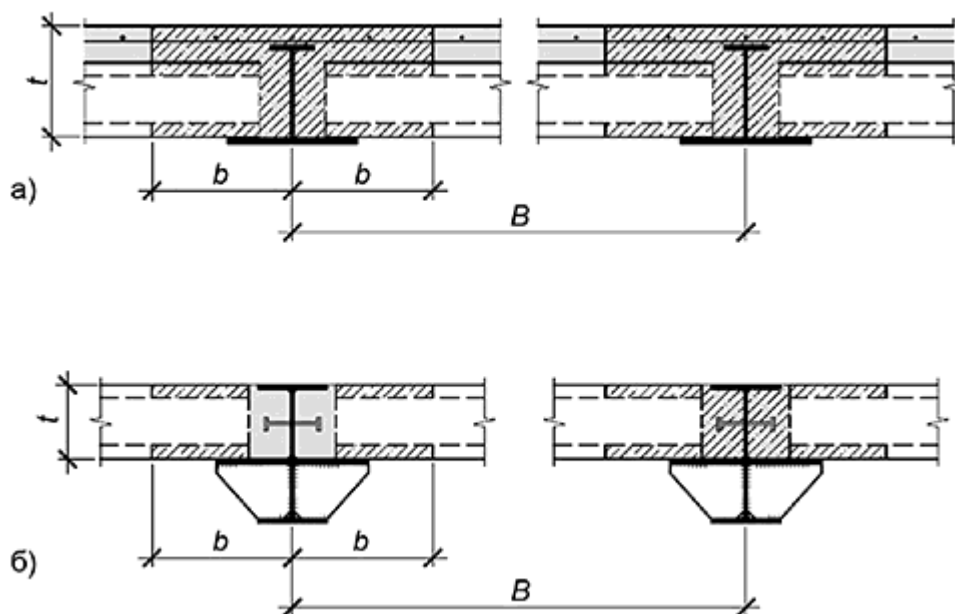
Рисунок 4.5, лист 2
