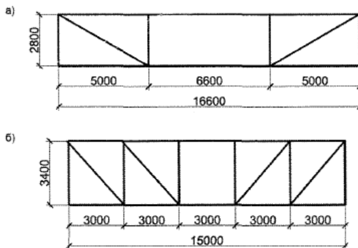
а) - схема фермы для общественного здания; б) - схема фермы для гаражей-стоянок
