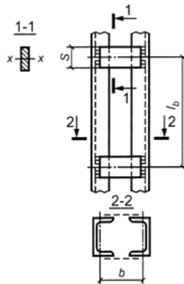
Рисунок 4 - Сквозной стержень с планками
