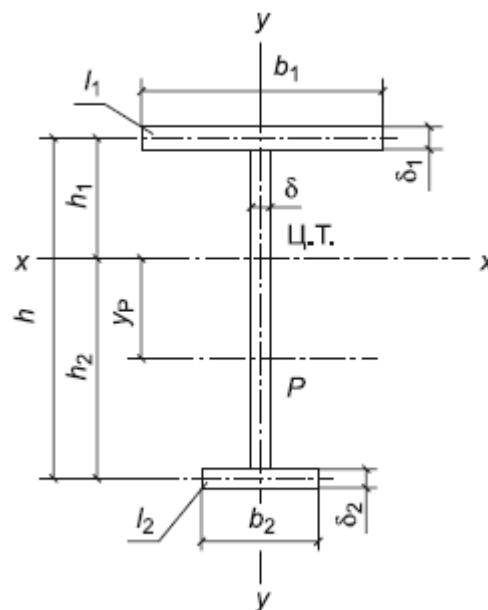
Рисунок Д.1 - Схема двутаврового сечения с одной осью симметрии
