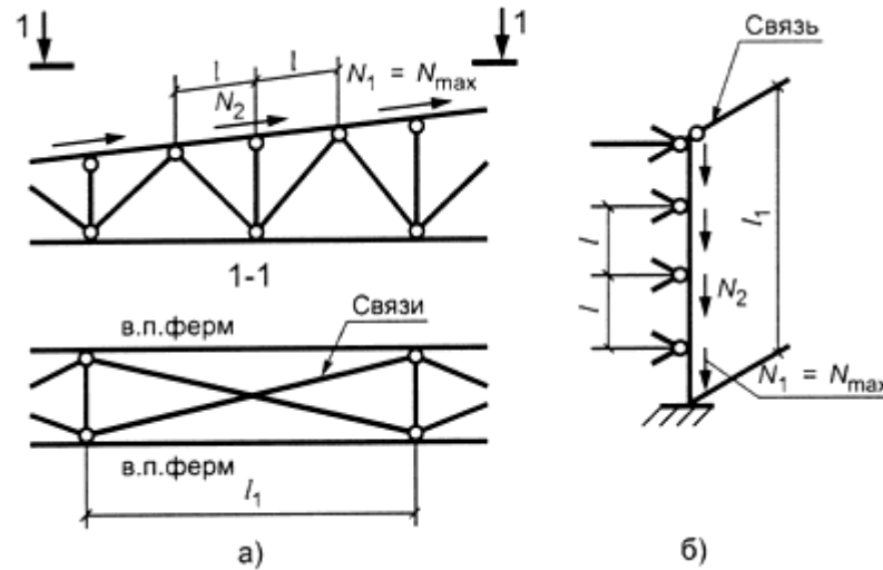
а - пояс фермы; б - ветвь колонны
