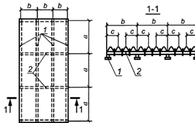
1 - продольные ребра; 2 - поперечные ребра
