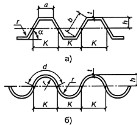
Рисунок 13 - Расчетная схема сжатого гофрированного листа
