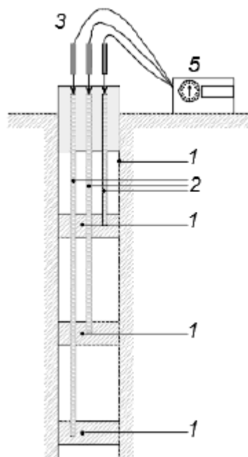
а) Стержневой экстензометр
