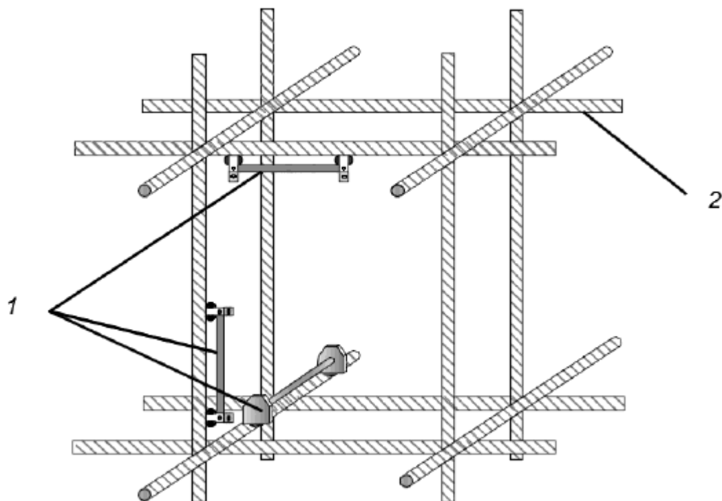
1 - накладные тензометрические датчики; 2 - арматурный каркас
