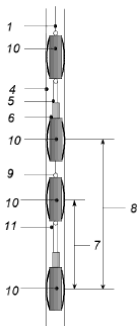
в) Стационарный инклинометр с измерительными модулями без направляющих роликов, модули не соединены в одну цепочку
