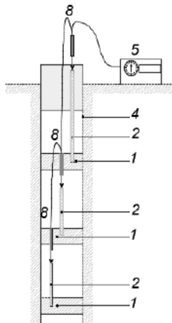
в) Звеньевой экстензометр
