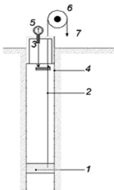
б) Проволочный экстензометр
