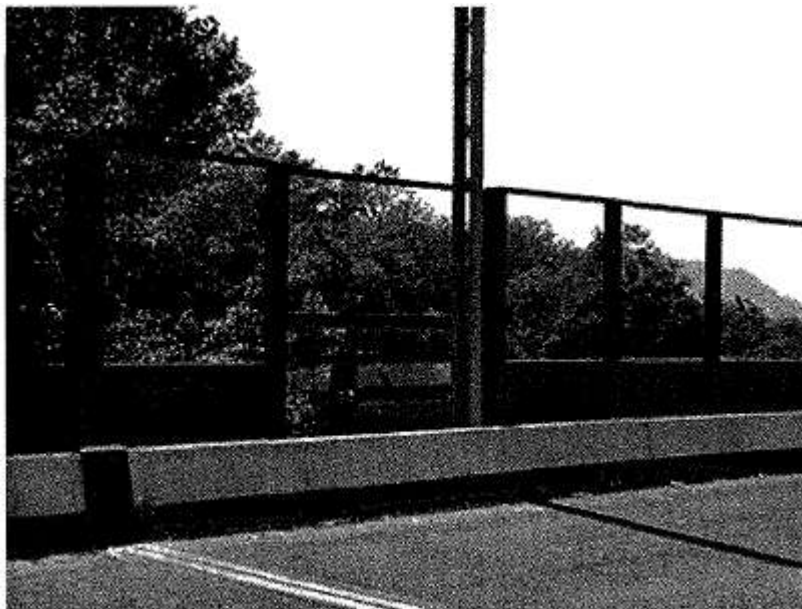
Рисунок А.5 - Нанесение силуэтов хищных птиц на прозрачные экраны
