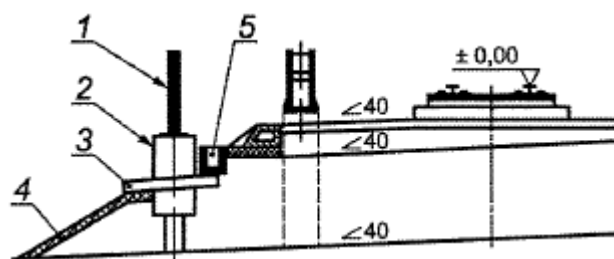
1 - ШЭ; 2 - низкий ростверк; 3 - поперечный водосбор; 4 - укрепленный откос; 5 - продольный водоотводный лоток
