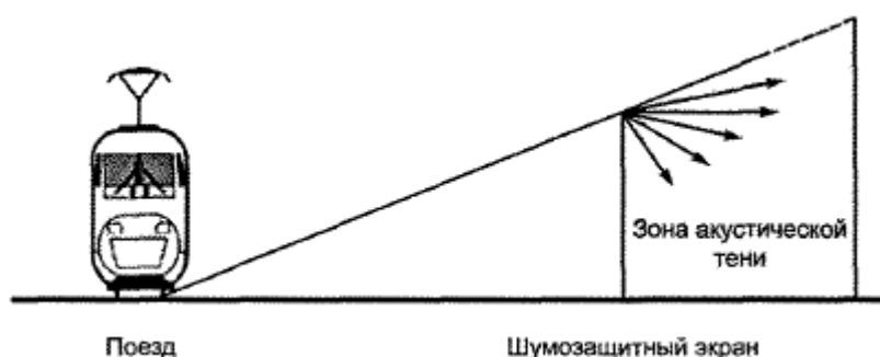
Рисунок 7.2 - Формирование зоны акустической тени
