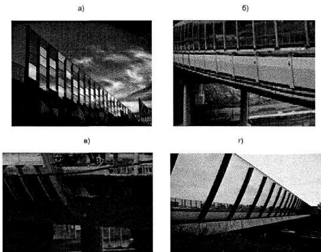
а - ШЭ, установленный на подпорной стене (стандартное крепление); б - ШЭ, закрепленный на закладной трубе, проходящей вдоль всего пролета эстакады (аналог выносной площадки); в - крепление точечных выносных площадок на металлические ребра жесткости пролета эстакады под стойки ШЭ (торцевое крепление); г - крепление стоек ШЭ на закладные элементы в железобетонном пролете моста (стандартное крепление)
