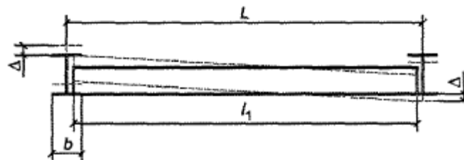
Рисунок 8.8 - Схема расчета предельных перемещений свободных концов несущих элементов 8.7.7 Стойки ШЭ классифицируют:
