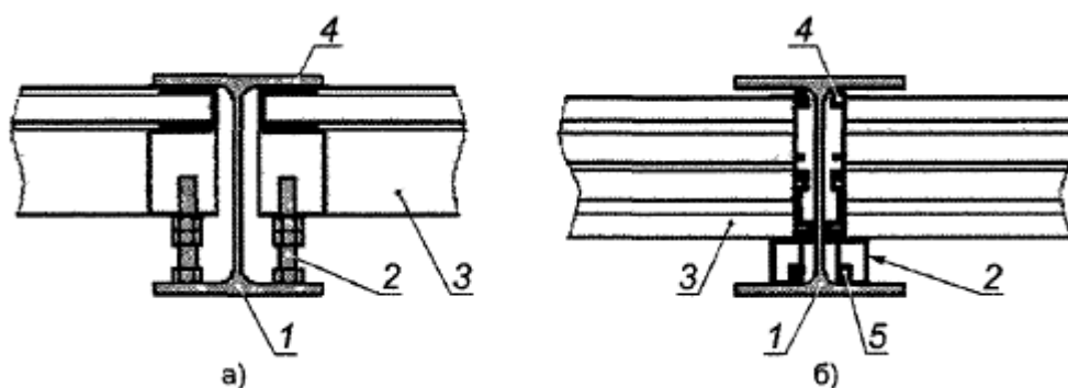
а - крепление панели распорным болтом внутри стойки; б - крепление панели специальным зажимом внутри стойки; 1 - стойка ШЭ; 2 - выбранный элемент крепления панели; 3 - панель ШЭ; 4, 5 - уплотнители
