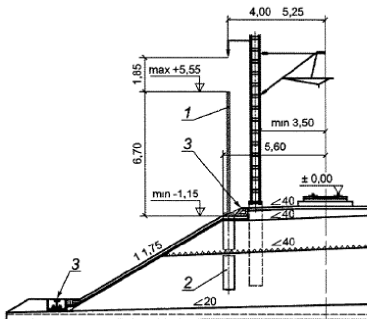
1 - ШЭ; 2 - фундамент ШЭ; 3 - лоток для кабелей
