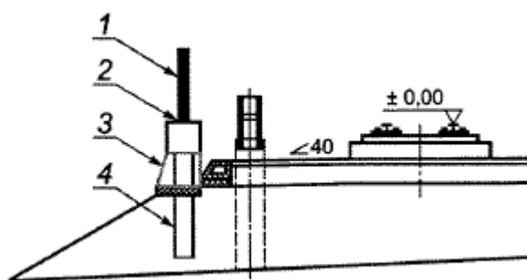
1 - ШЭ; 2 - высокий ростверк; 3 - дренирующий материал; 4 - свайный фундамент
