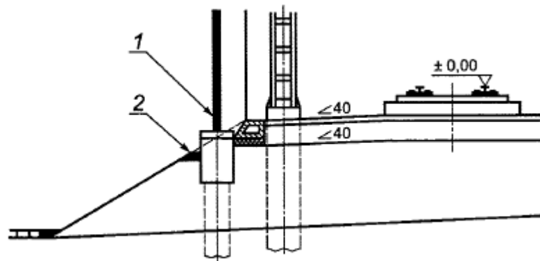
1 - ШЭ; 2 - свайный фундамент без ростверка
