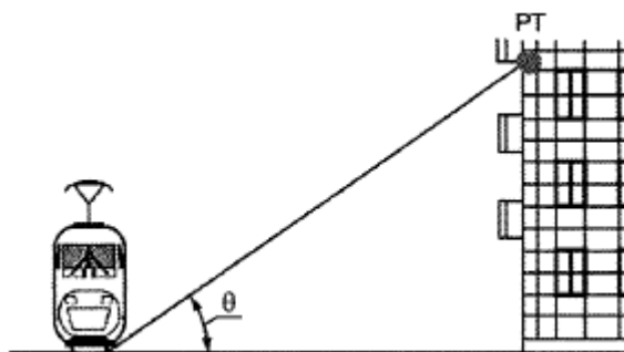
Рисунок 6.3 - Определение угла \theta направленности шума качения, излучаемого ходовой частью поезда
