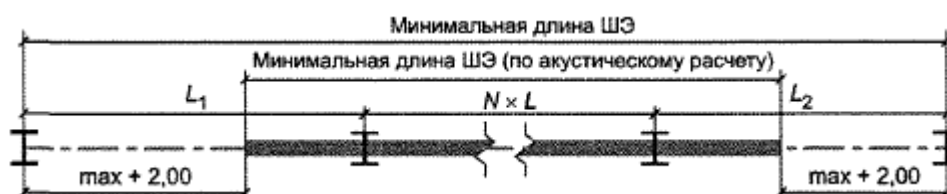
Рисунок 8.1 - Определение максимальной и минимальной длин шумозащитного экрана
