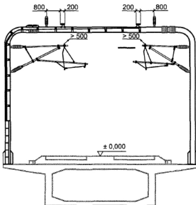
Рисунок 8.10 - Выполнение тоннельных галерей и совмещение конструкций
