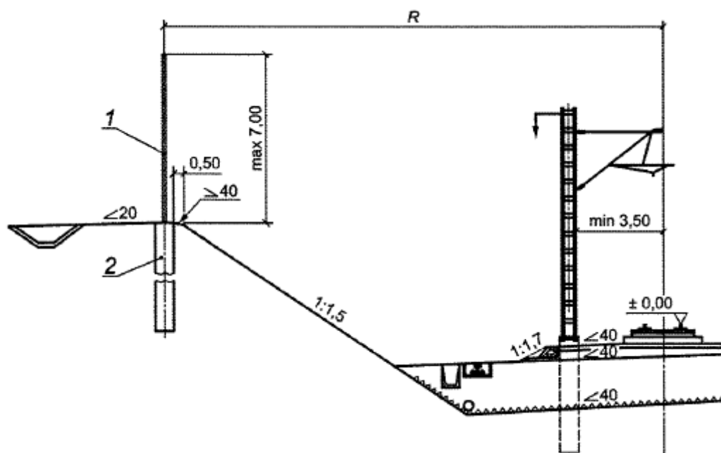
Рисунок 8.22 - Пример установки шумозащитного экрана в пределах откоса земляного полотна
