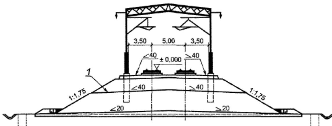
1 - раздельный слой из геотекстиля
