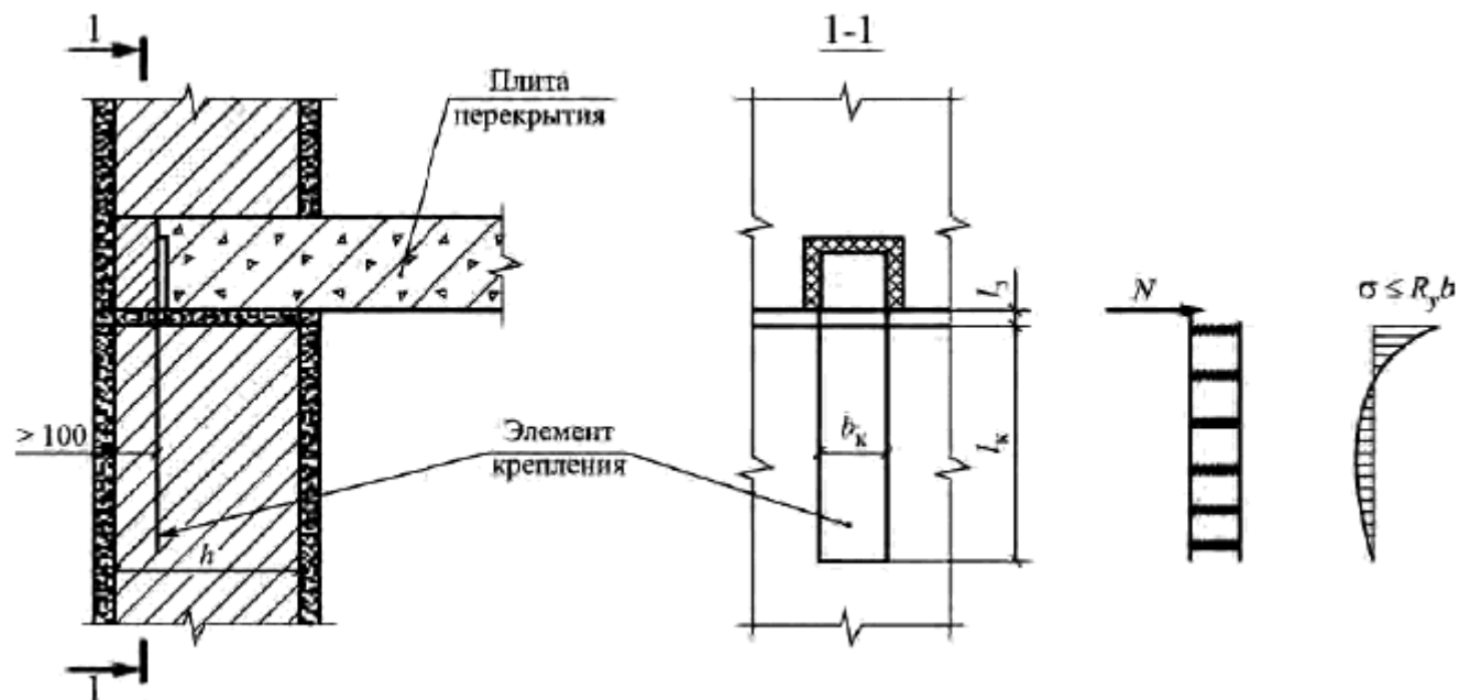
Рисунок 7.2 - К расчету полистиролбетонных стен
