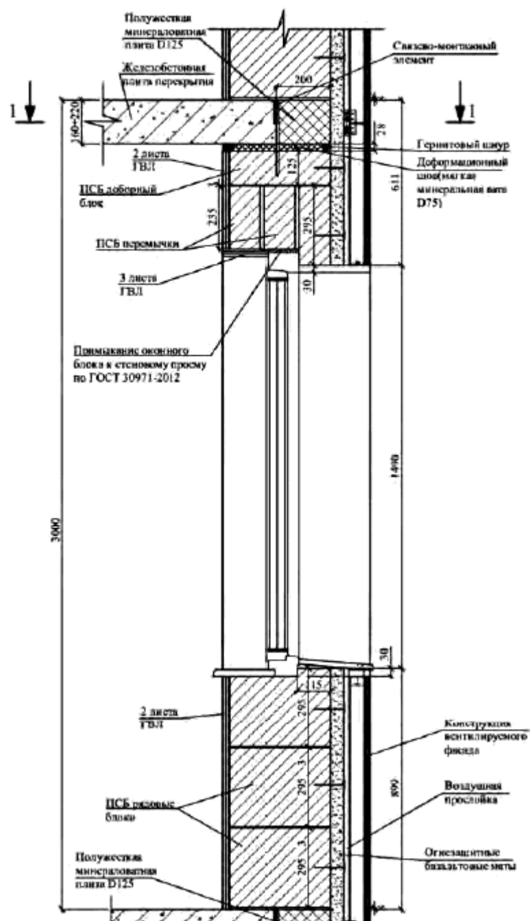
Разрез по термовкладышу в перекрытии
