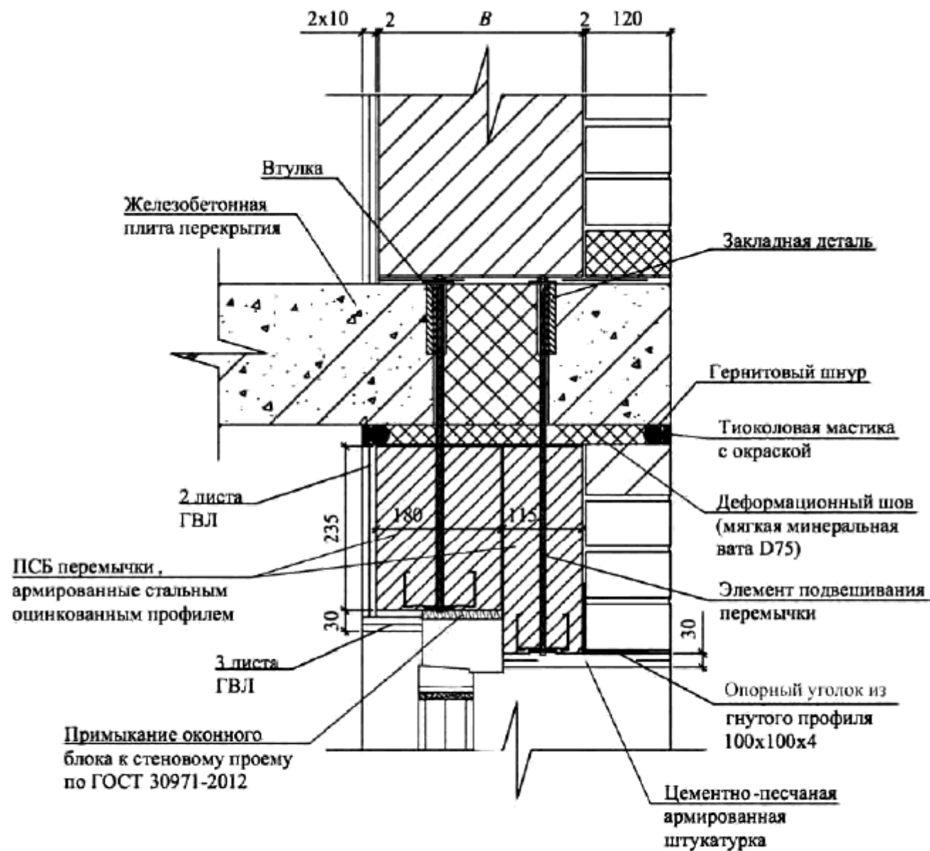
План-схема расположения элементов подвешивания перемычек
