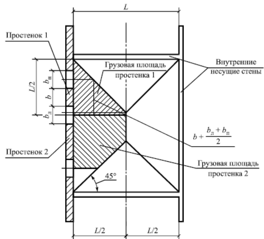
Рисунок 7.8 - Схема определения грузовой площади стены
