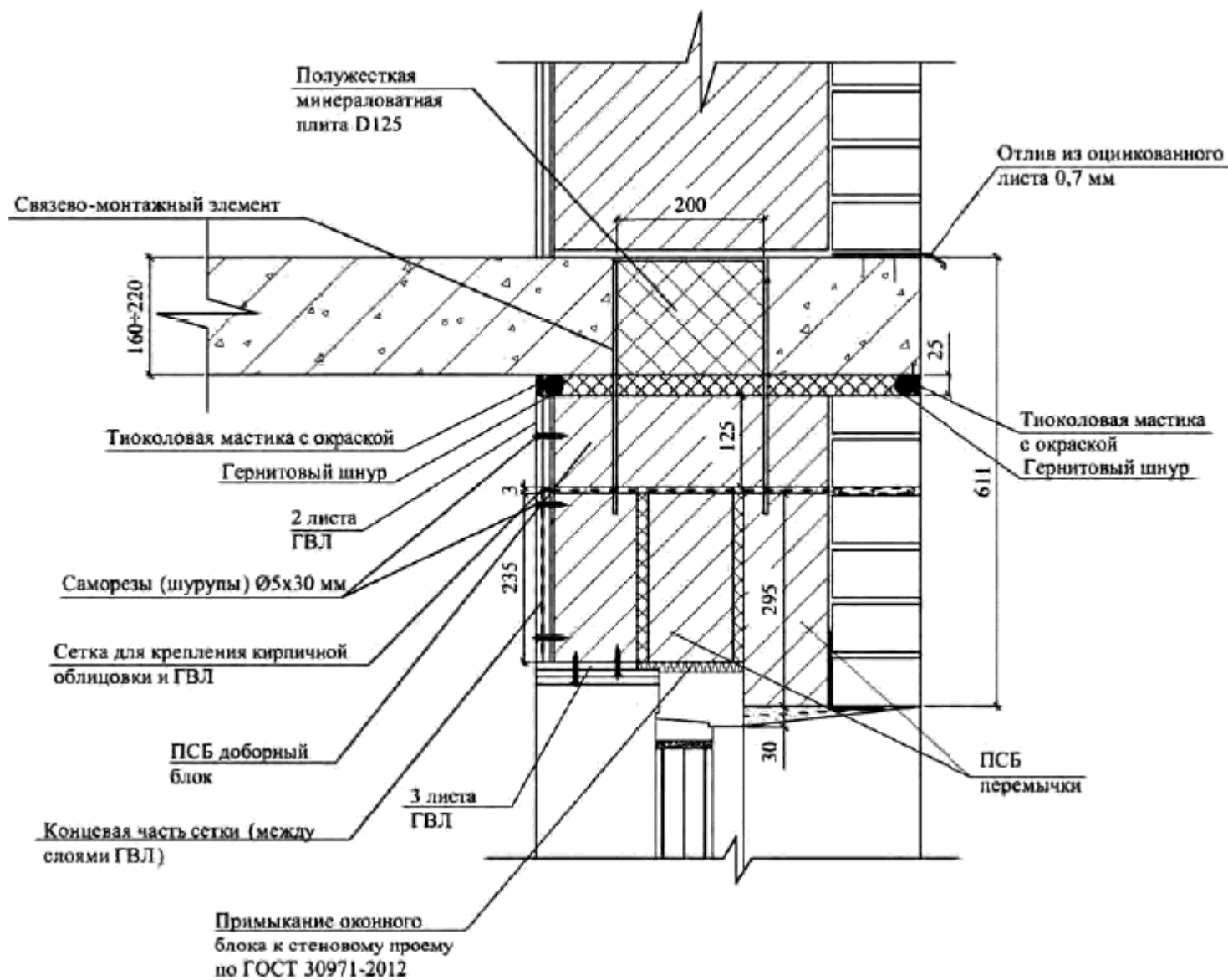
Рисунок 6.18 - Крепление ГВЛ к кладке из ПСБ блоков с использованием штукатурной сетки
