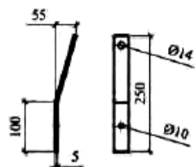
Опорная пластина для верхних кронштейнов
