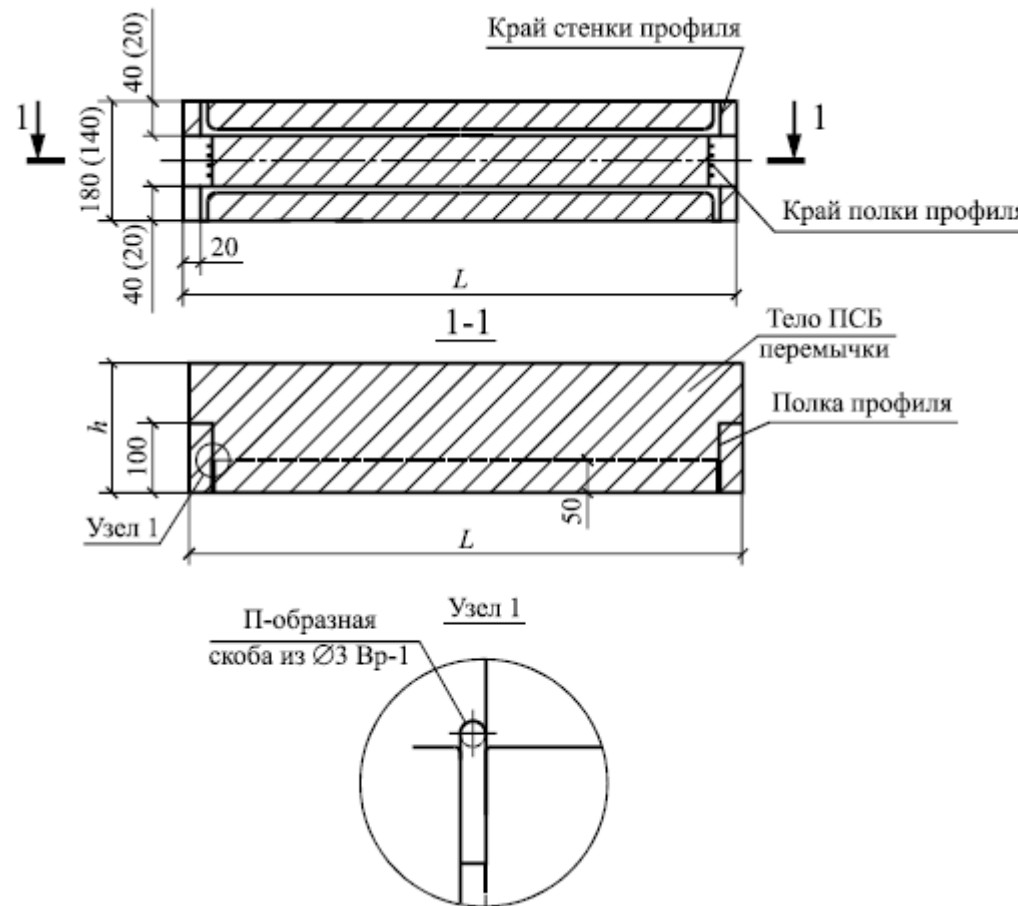
Рисунок 7.7 - Конструкция перемычки шириной 180 (140) мм с анкеровкой стального профиля по ее торцам Условие прочности нормальных сечений изгибаемого элемента записывают в виде
