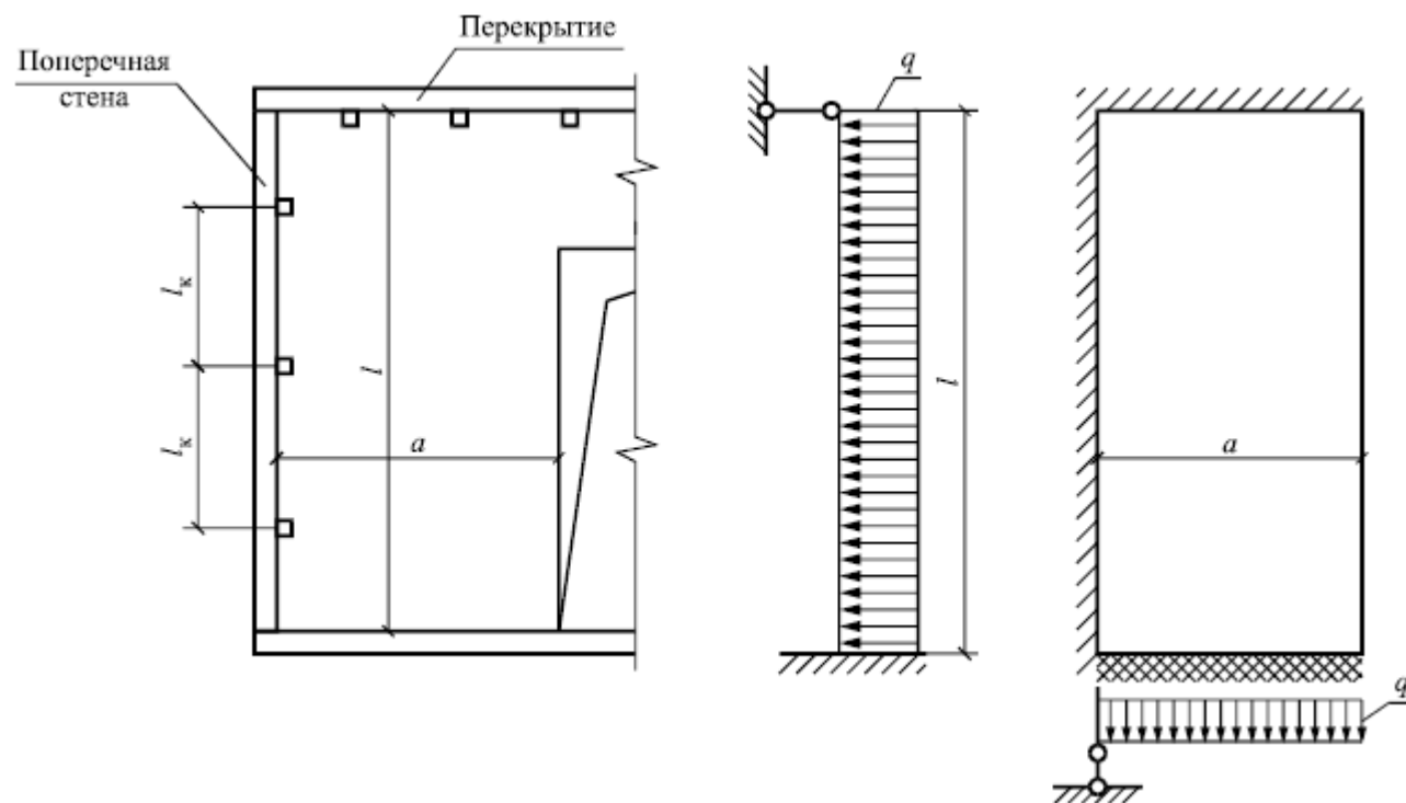
Рисунок 7.3 - К расчету силы N
