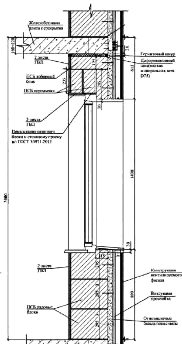
Разрез по шпонке в перекрытии
