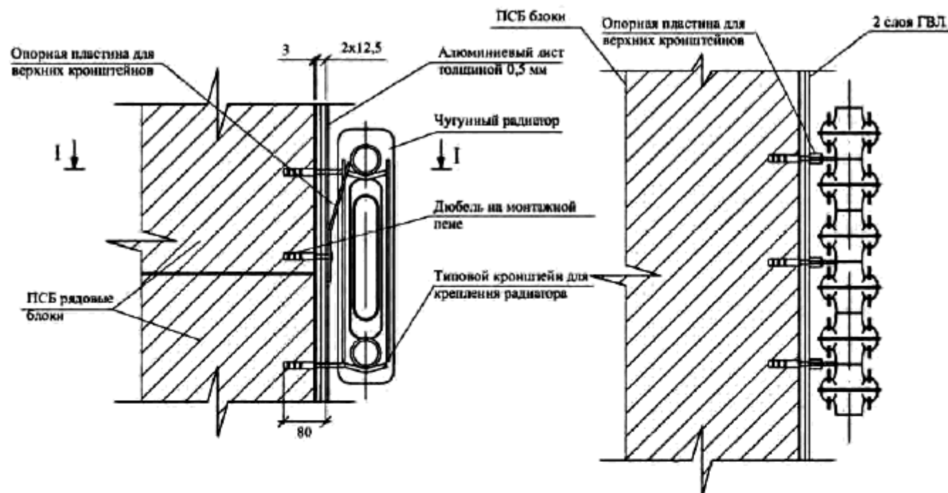
Кронштейн
