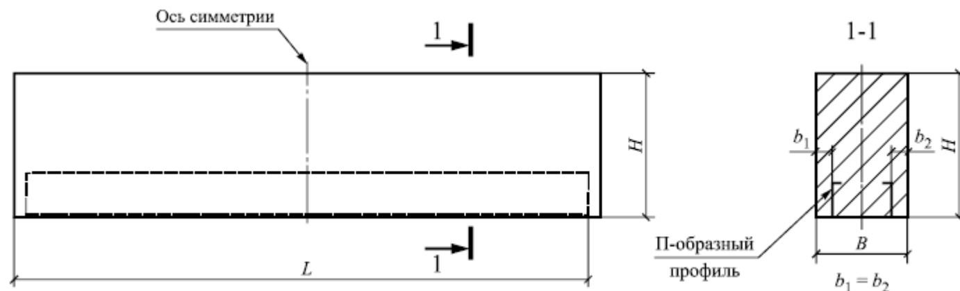
Рисунок 4.2 - Полистиролбетонная перемычка, армированная П-образным стальным оцинкованным профилем
