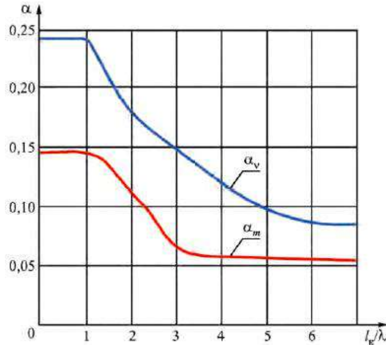
Рисунок 7.4 - График зависимости \alpha_v и \alpha_m от приведенной длины балки При креплении стены к верхнему перекрытию силу N принимают равной
