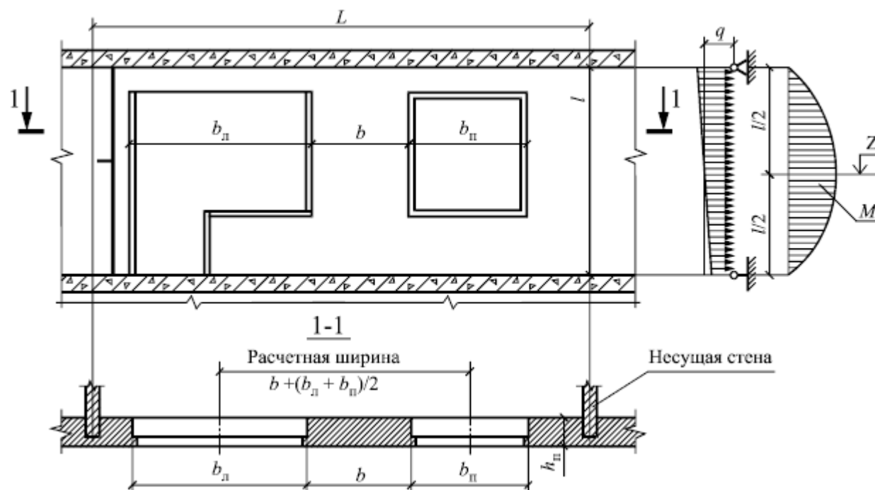
Рисунок 7.1 - К расчету простенка на ветровую нагрузку
