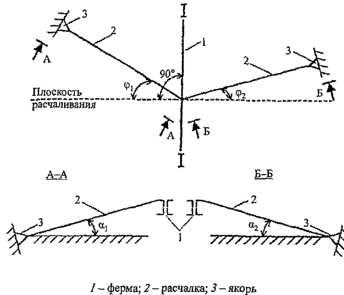
Рисунок К.2 – Схема раскрепления ферм расчалками
