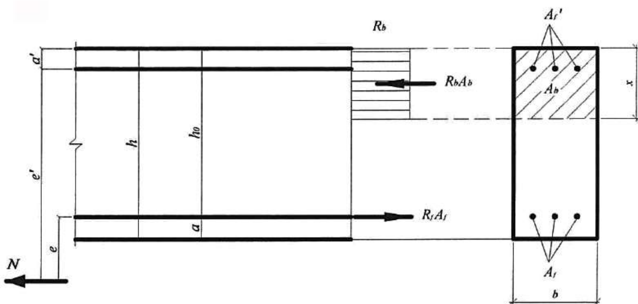
Рисунок 4 - Схема усилий и эпюра напряжений в сечении, нормальном к продольной оси внецентренно растянутой конструкции, при расчете ее по прочности при приложении продольной силы N между равнодействующими усилий в арматуре (а) и за пределами расстояния между равнодействующими усилий в арматуре (б)
