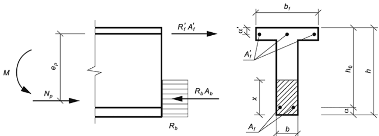
Рисунок 9* - Схема усилий и эпюра напряжений в сечении, нормальном к продольной оси изгибаемой предварительно напряженной конструкции при ее расчете по прочности в стадии обжатия
