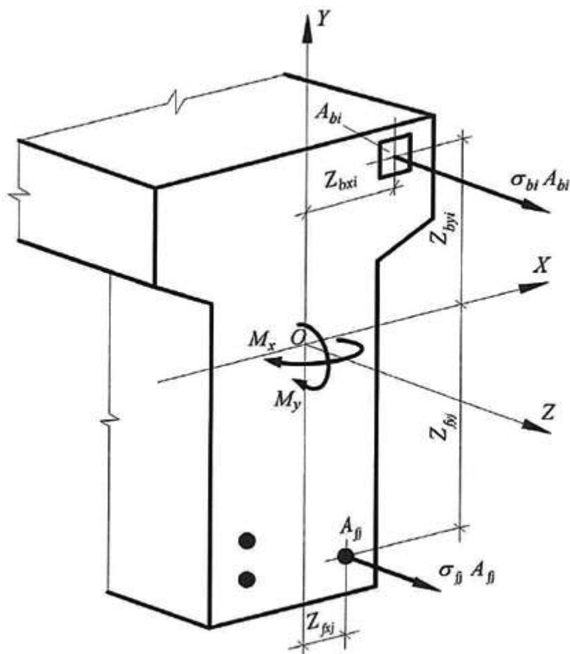
Рисунок 5 - Расчетная схема нормального сечения конструкции Расчет нормальных сечений конструкций по прочности производят из условий:
