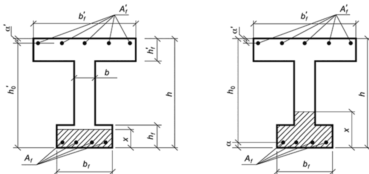
Рисунок 9а* - Положение границы сжатой зоны в сечении изгибаемой предварительно напряженной конструкции с полкой в сжатой зоне при ее расчете по прочности в стадии обжатия
