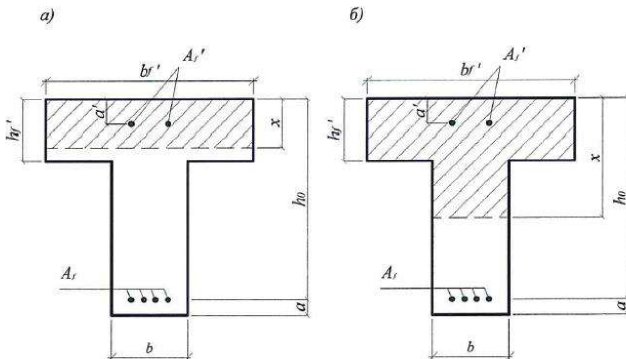
Рисунок 2 - Положение границы сжатой зоны в сечении изгибаемой конструкции Значение b'_f , вводимое в расчет, принимают по СП 63.13330.
