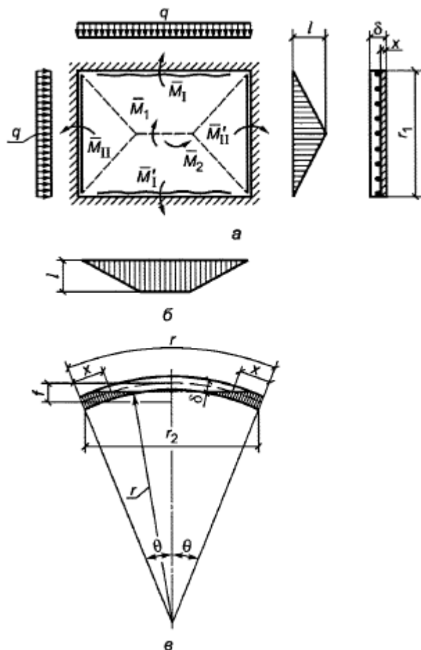
а - схема изло, б - перемещения панели в предельной стадии, в - сечение по криволинейному контуру панели
