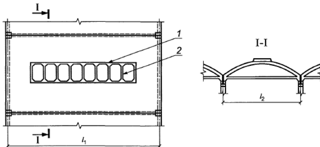
1 - рамка окаймления фонарного отверстия, 2 - распорка
