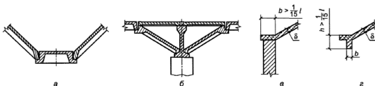
а - п-образных, б - двутавровых с плитами поверху, в - крайних, г - при опирании на колонны
