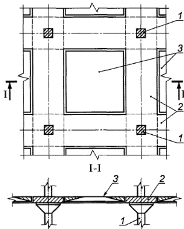
1 - колонна, 2 - надколонные плиты, 3 - вспарушенные панели
