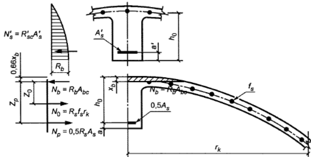
Рисунок 11.19 - Схема взаимодействия усилий в радиальном сечении оболочек Для наиболее распространенного случая ребер трапецевидного сечения предельный момент в кольцевых сечениях \overline{M}_{rh} определяют по формуле
