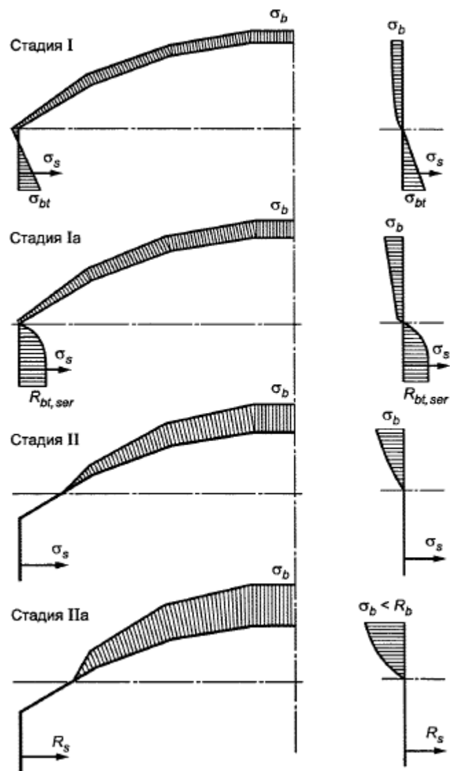
Рисунок 9.7 - Стадии напряженного состояния поперечных сечений оболочки (складки)
