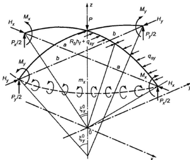
Рисунок 11.20 - Схема взаимодействия усилий в зоне приложения сосредоточенной нагрузки
