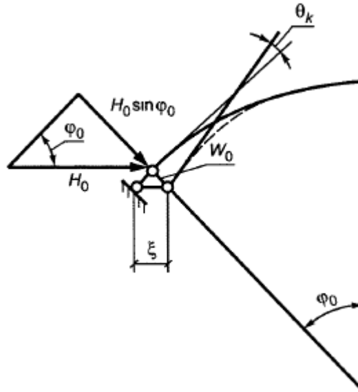
Рисунок 10.3 - Перемещения края оболочки, вызванные радиальным распором H_0
