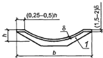
1 - ребра по поперечным краям элементов
