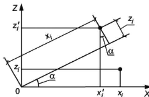
Рисунок 17.4 - Преобразование координат
