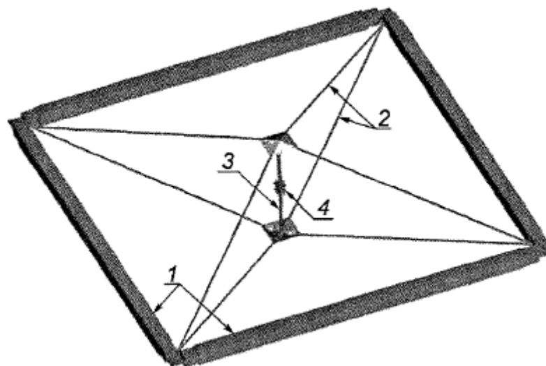
1 - контурный элемент; 2 - наклонный стержень; 3 - центральная стойка; 4 - домкрат
