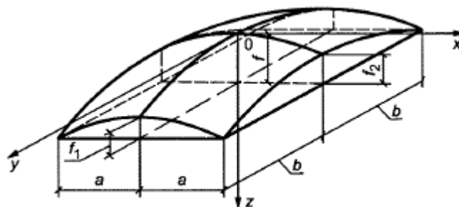
Рисунок 11.1 - Схема оболочки положительной гауссовой кривизны
