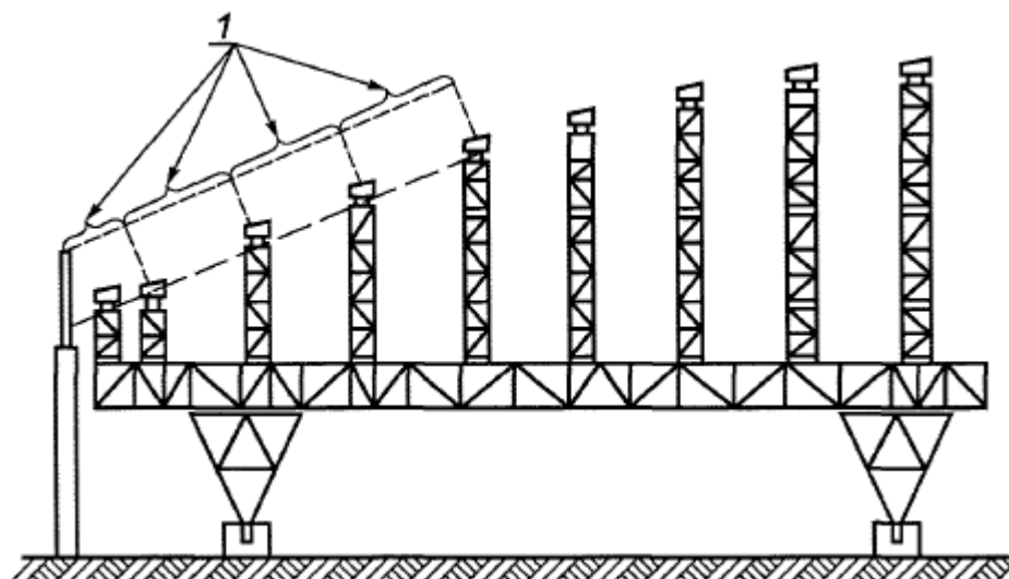
1 - укрупненные монтажные блоки
