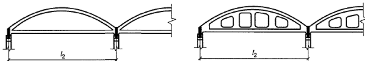
Рисунок 9.11 - Диафрагмы цилиндрических оболочек
