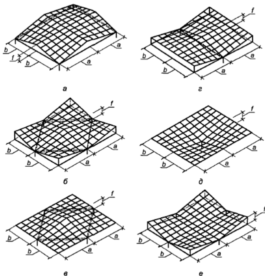
а-е - варианты формы покрытий
