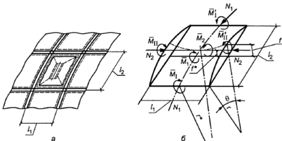
Рисунок 11.15 - Расчетная схема плиты ребристой цилиндрической панели сборной оболочки, расположенной в приконтурной зоне
