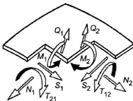
Рисунок 11.5 - Схема усилий в пологих оболочках
