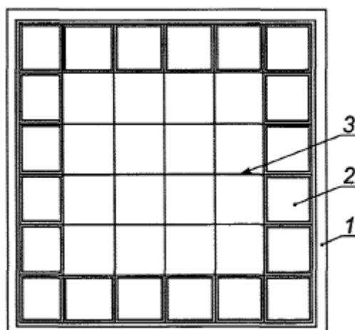
1 - опорный контур; 2 - плита; 3 - ванты
