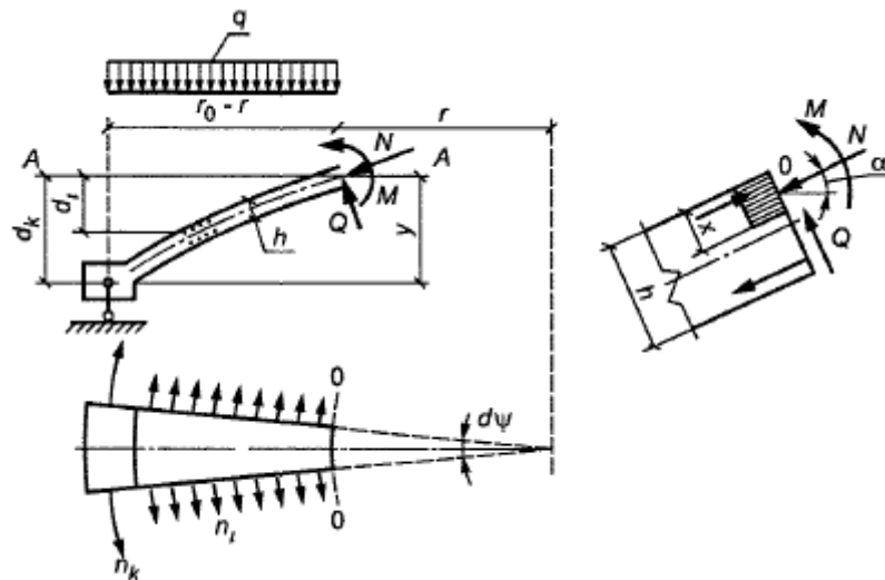
Рисунок 10.6 - Схема взаимодействия усилий в куполе в предельном состоянии Предельное усилие на единицу длины в кольцевых стержнях поля оболочки n определяется по формуле
