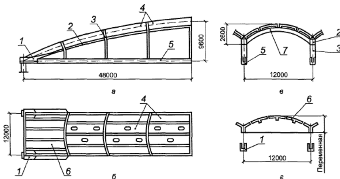
а - продольный разрез по своду, б - план раскладки плит, в - поперечный разрез по средней зоне, г - то же по опорной зоне, 1 - опорный блок, 2 - бортовые элементы, 3 - стальная подвеска, 4 - средняя плита с отверстиями, 5 - блок затяжки, 6 - плита опорной зоны, 7 - балка диафрагмы
