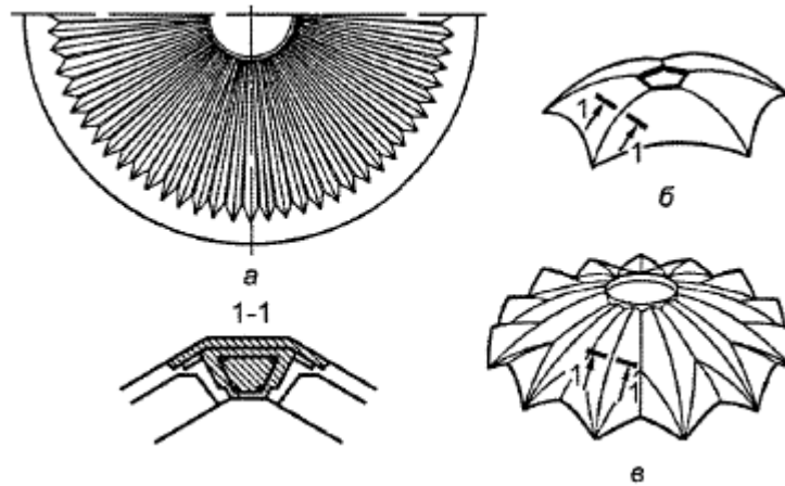
а - складчатый купол; б, в - сопряженные купольные оболочки
