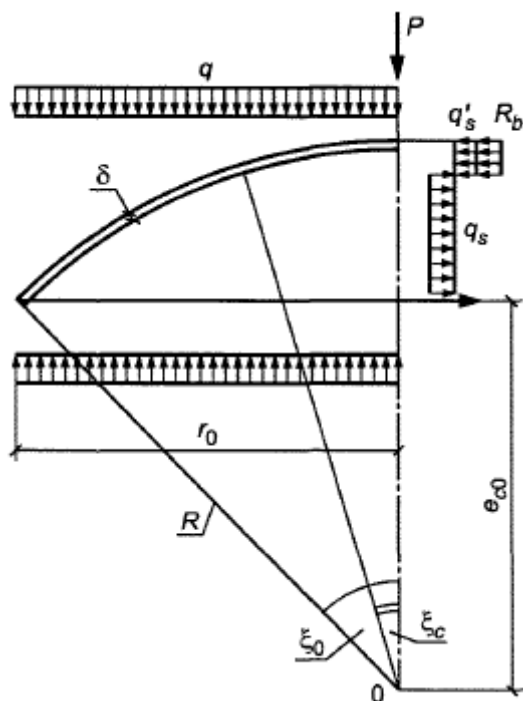
Рисунок 10.8 - К расчету купола по "балочной" схеме
