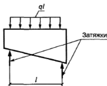
Рисунок 7.7 - Расчетная схема опорной панели
