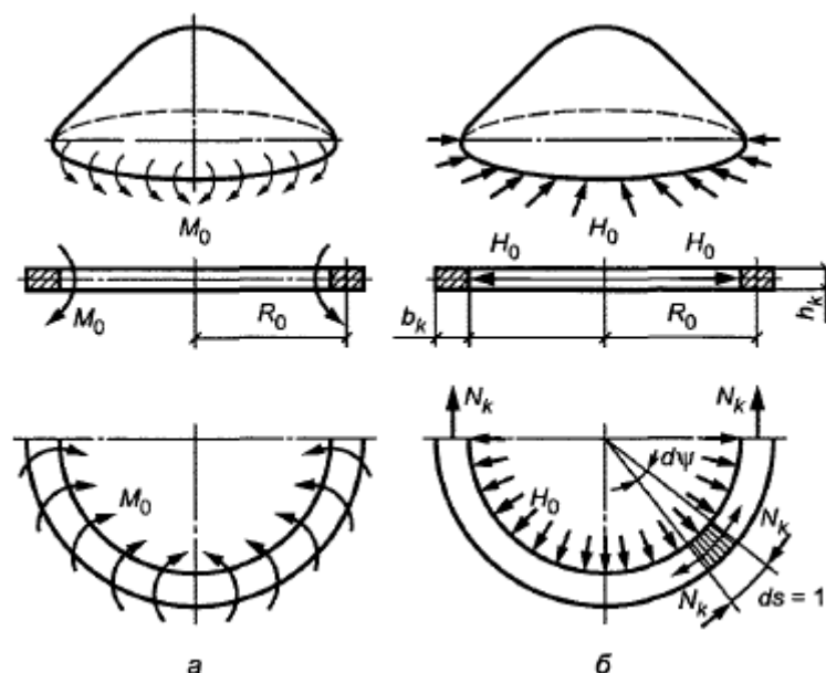
а - момент, б - распор
