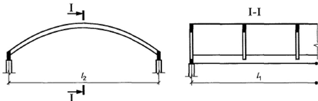
Рисунок 9.9 - Ребристая оболочка
