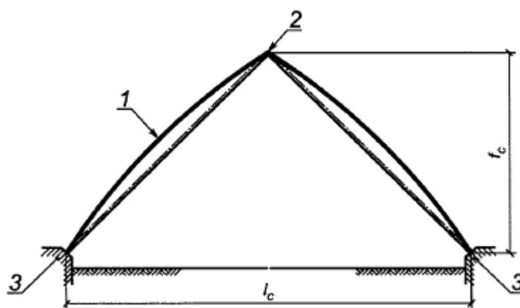
Рисунок 14.10 - Конструктивная схема сегментного свода для покрытий, опирающегося на продольные балки каркаса здания
