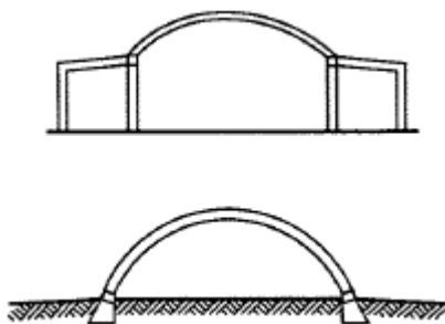
Рисунок 7.2 - Своды без затяжек
