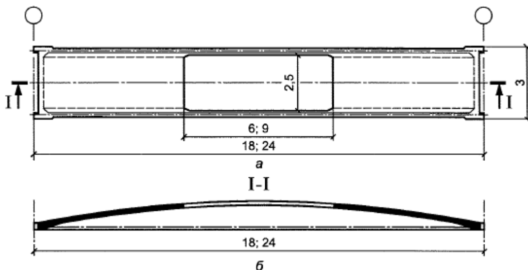
а - план, б - продольный разрез по оси панели
