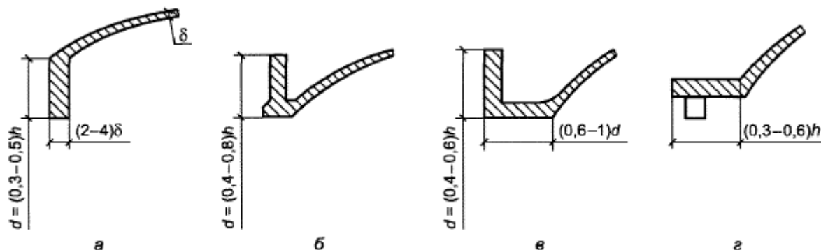
Рисунок 9.10 - Бортовые элементы
