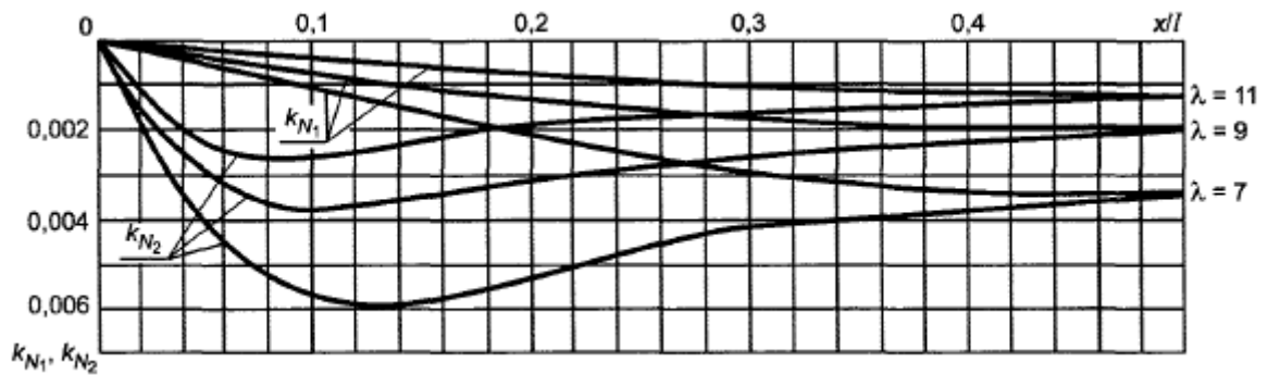
Рисунок 11.6 - Графики коэффициентов k_{N1} , k_{N2}
