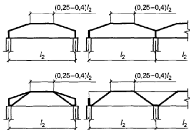
Рисунок 9.2 - Складчатые оболочки с различными типами бортовых элементов
