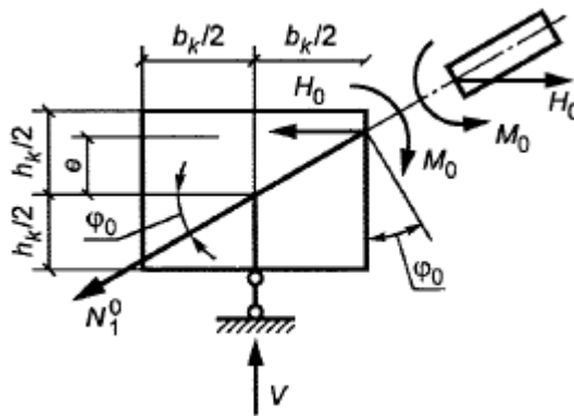
Рисунок 10.2 - Расчетная схема узла сопряжения опорного кольца и оболочки купола 10.3. Перемещения края оболочки, вызванные радиальным распором H_0 , приведены на рисунке
