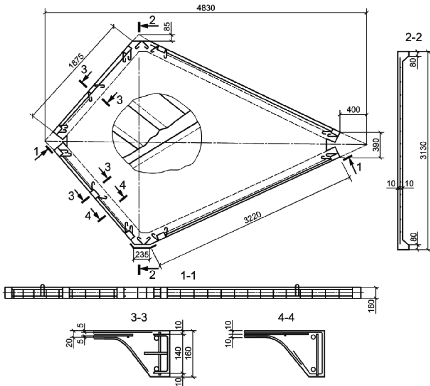
Рисунок 17.7 - Принципиальное решение армирования ромбического элемента
