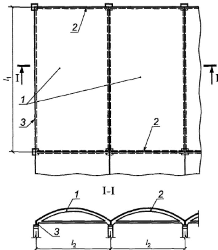
1 - плита оболочки; 2 - диафрагма; 3 - бортовой элемент
