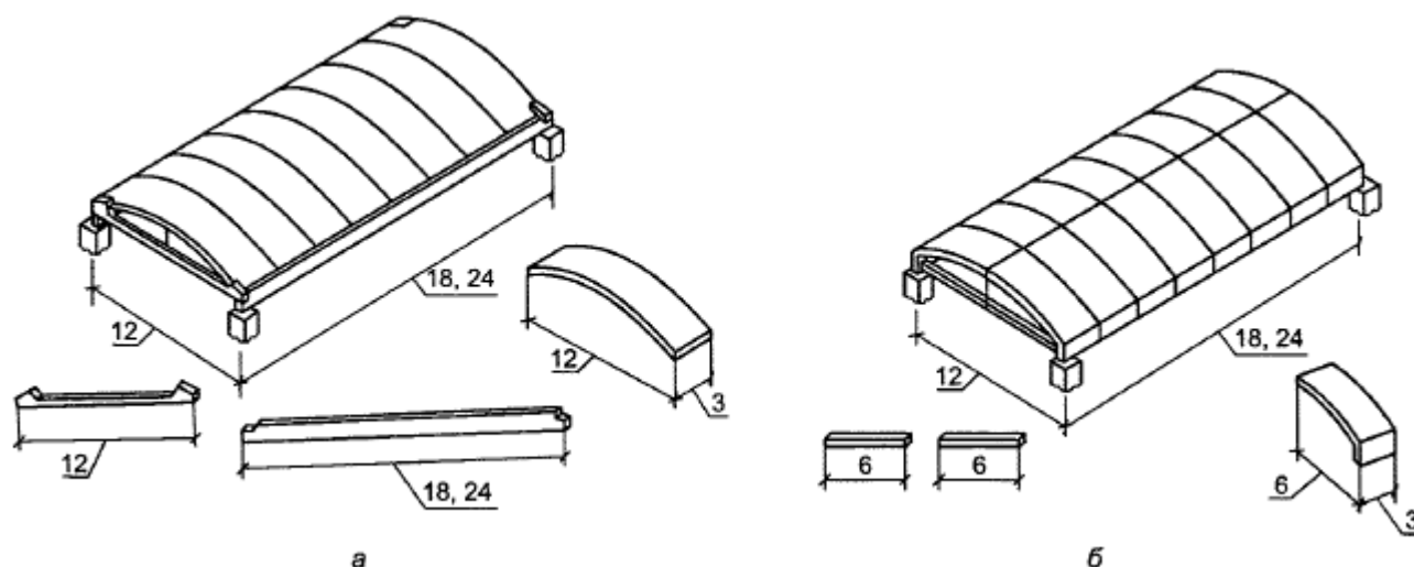
а - из бортовых балок, криволинейных ребристых панелей и затяжек диафрагм, б - из криволинейных ребристых панелей с бортовым элементом и затяжек диафрагм
