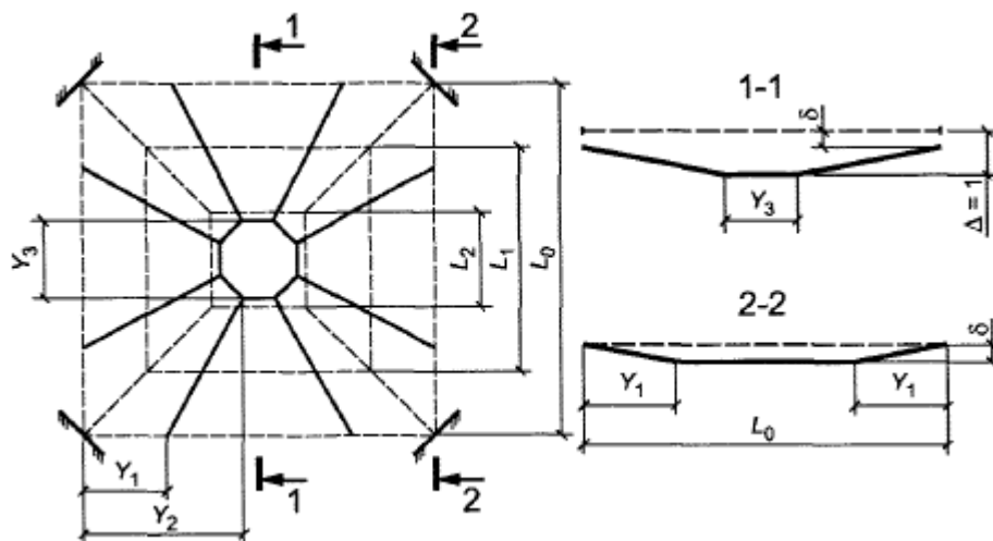
Рисунок 16.3 - Девятидисксовая схема излома
