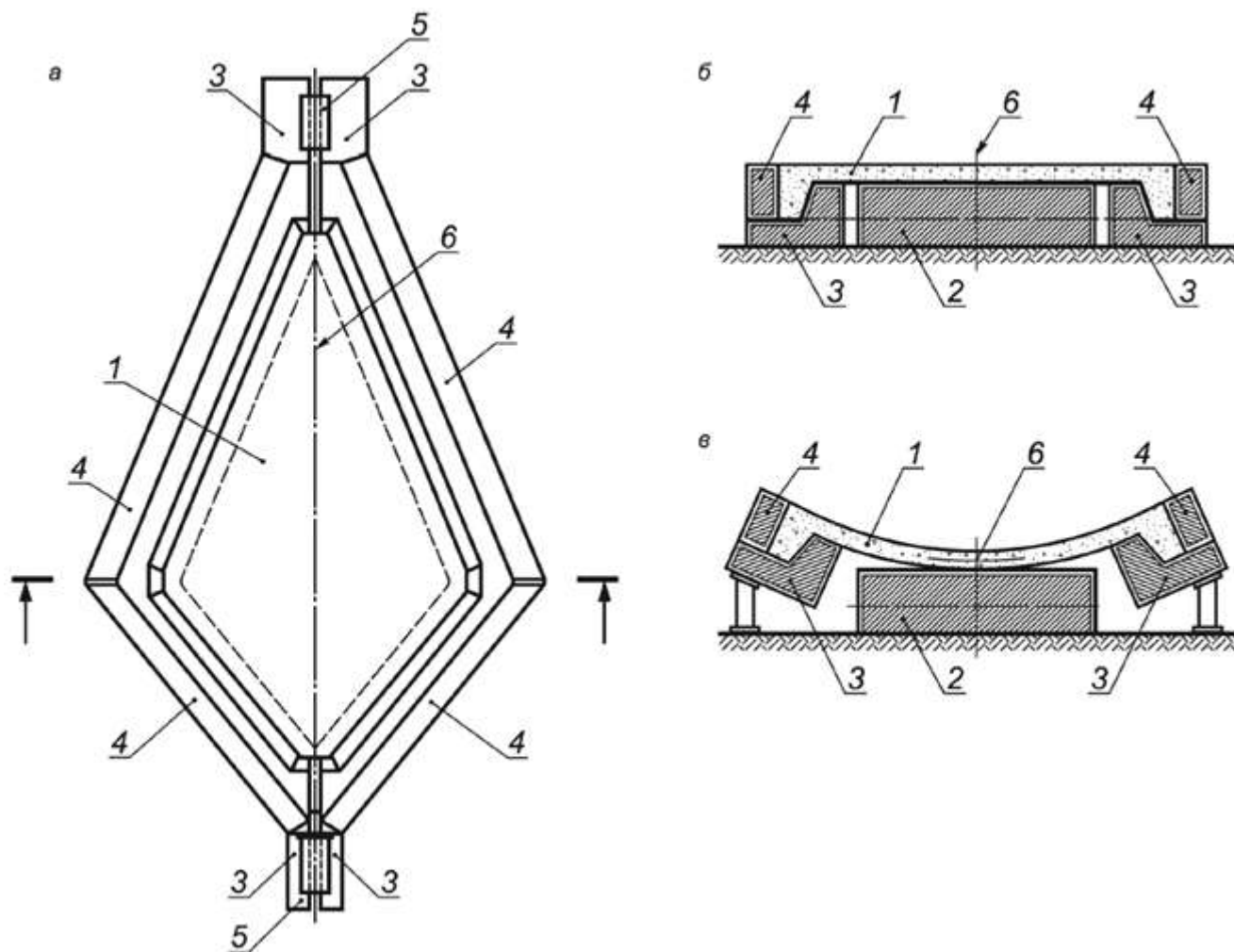
а - план; б, в - поперечный разрез соответственно в исходном и согнутом состоянии; 1 - гибкий поддон; 2 - жесткий поддон; 3 - элемент жесткой рамы; 4 - откидной борт; 5 - соосные шарниры; 6 - ось шарниров
