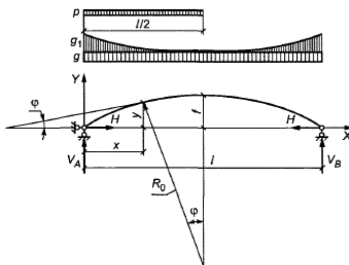
Рисунок 7.4 - Расчетная схема свода
