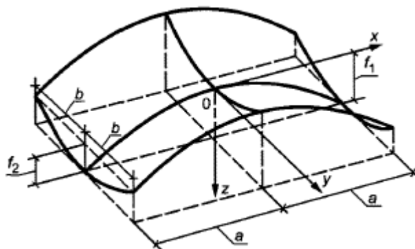
Рисунок 12.1 - Гиперболический параболоид
