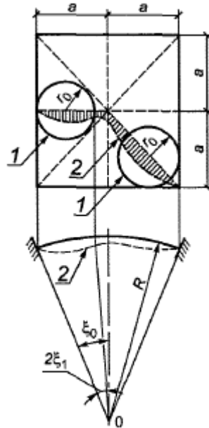
1 - вероятные места образования вмятин; 2 - кривая прогибов
