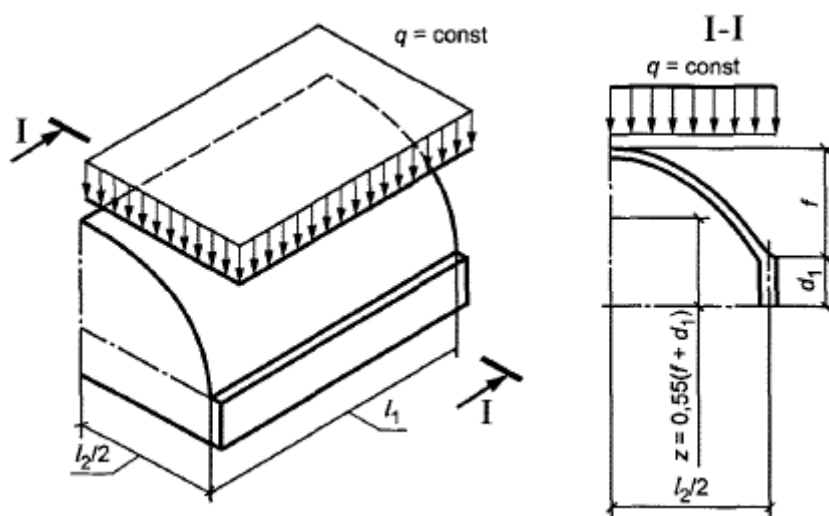
Рисунок 9.16 - К расчету бортового элемента короткой цилиндрической оболочки
