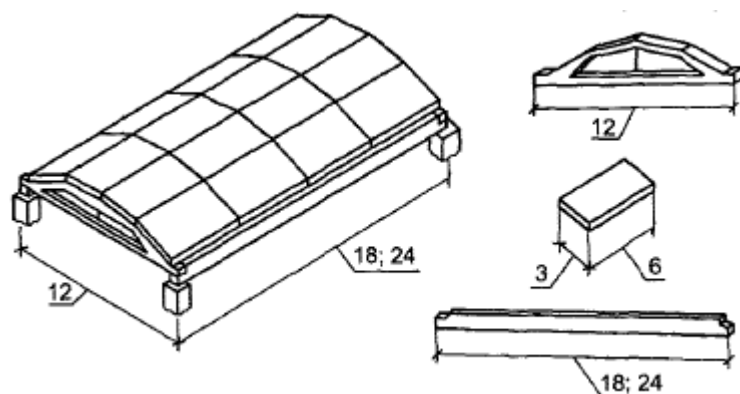
Рисунок 9.14 - Складчатые оболочки из бортовых балок, арок-диафрагм и плоских ребристых или гладких плит
