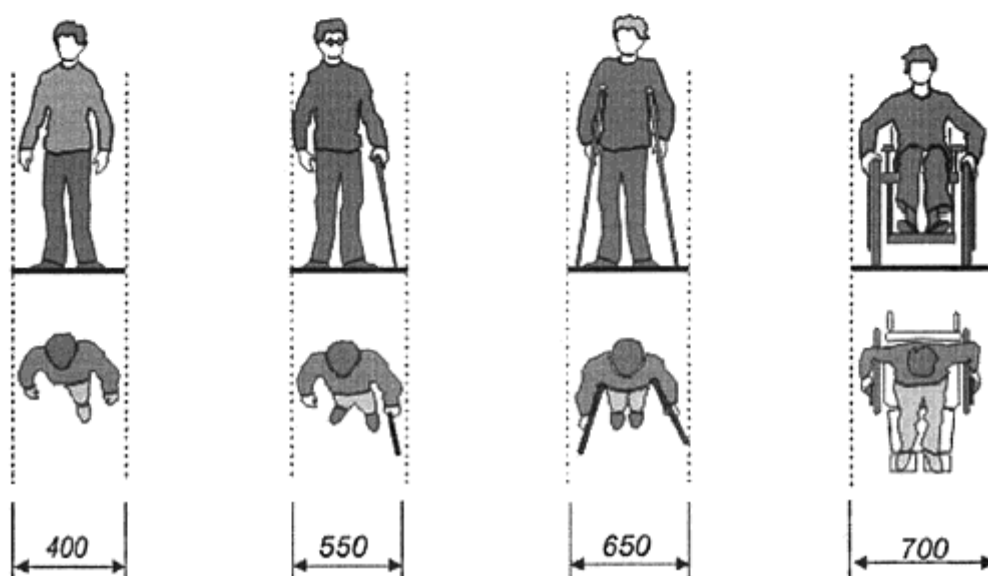
Минимальные габариты полосы движения для детей-инвалидов.
