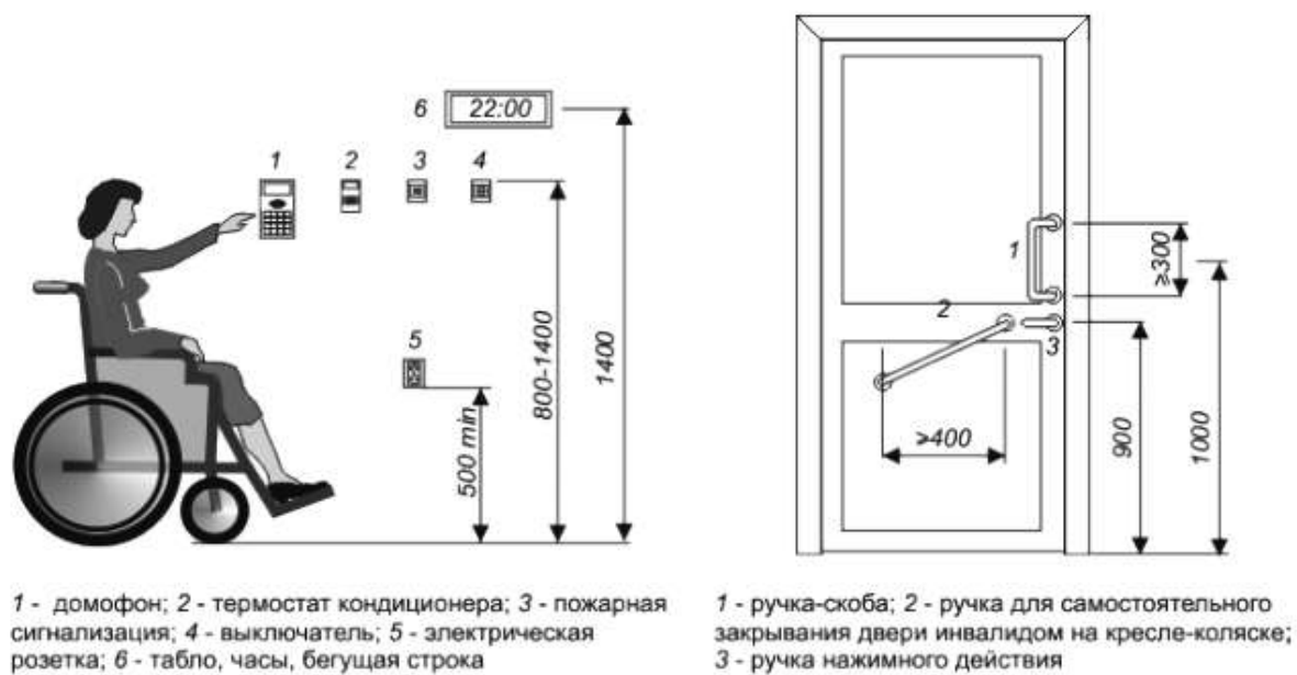
Рисунок Г.6 - Досягаемость оборудования
