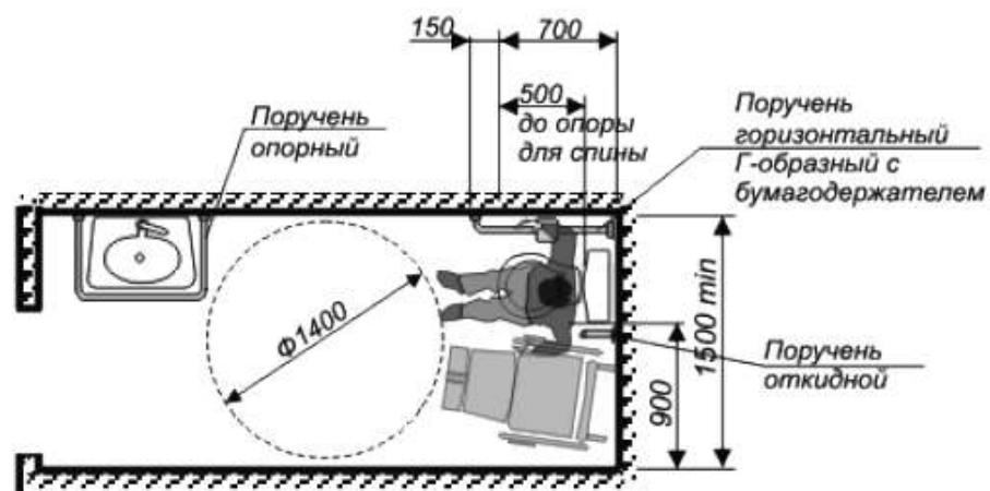
Рисунок Г.12 - Примеры оборудования совмещенного санитарного узла
