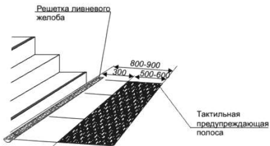
Параметры тактильных контрастных полос на ступенях
