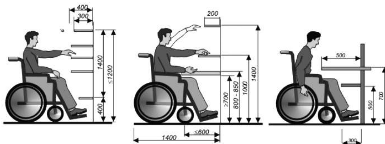
Рисунок Г.1 - Зоны досягаемости инвалидов на кресле-коляске
