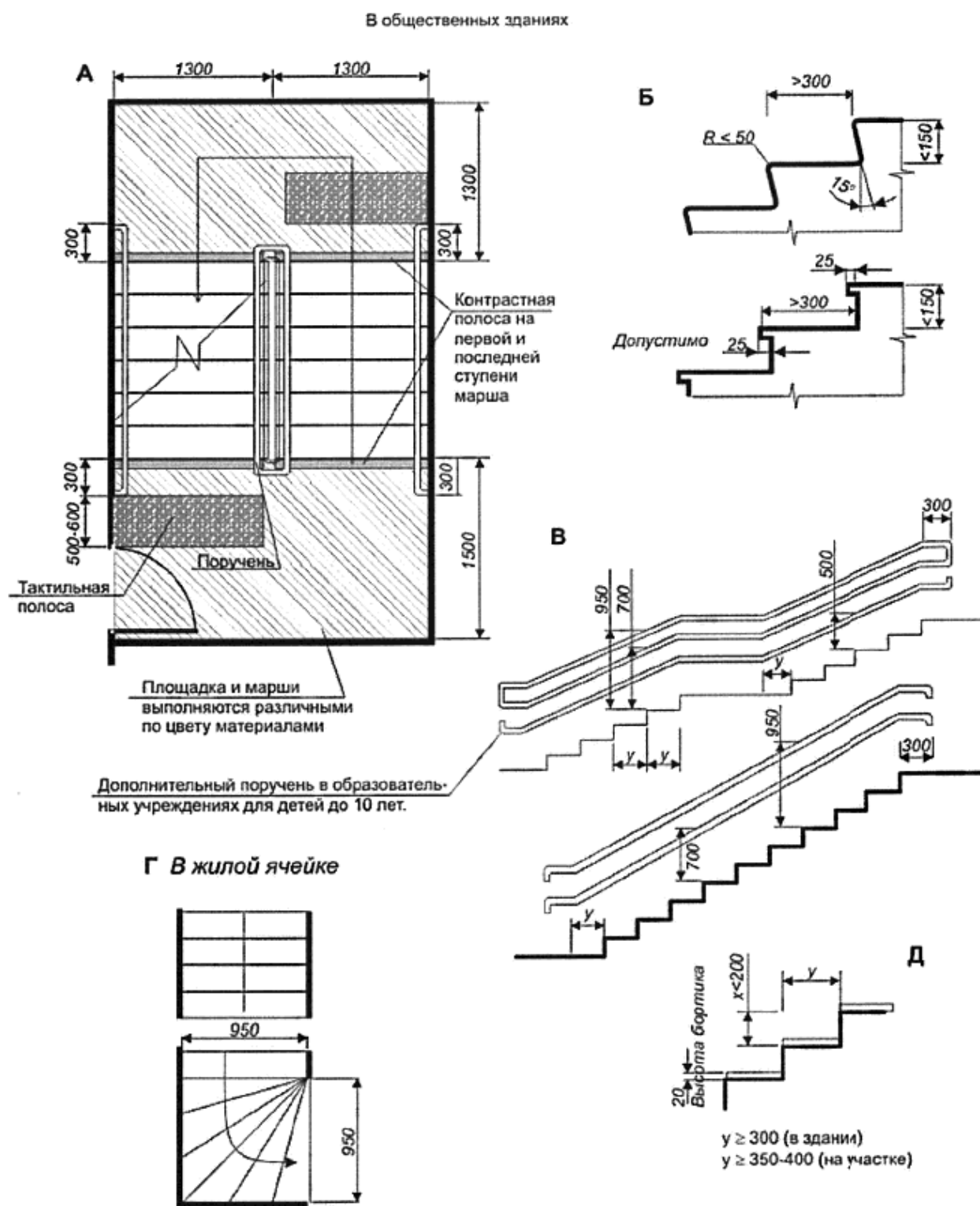
Рисунок В.22 - Предупреждающие контрастные и тактильные полосы
