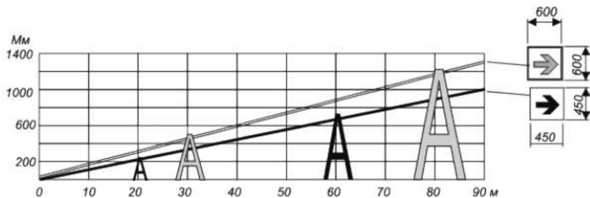
Рисунок Г.14 - Обеспечение фронта видимости
