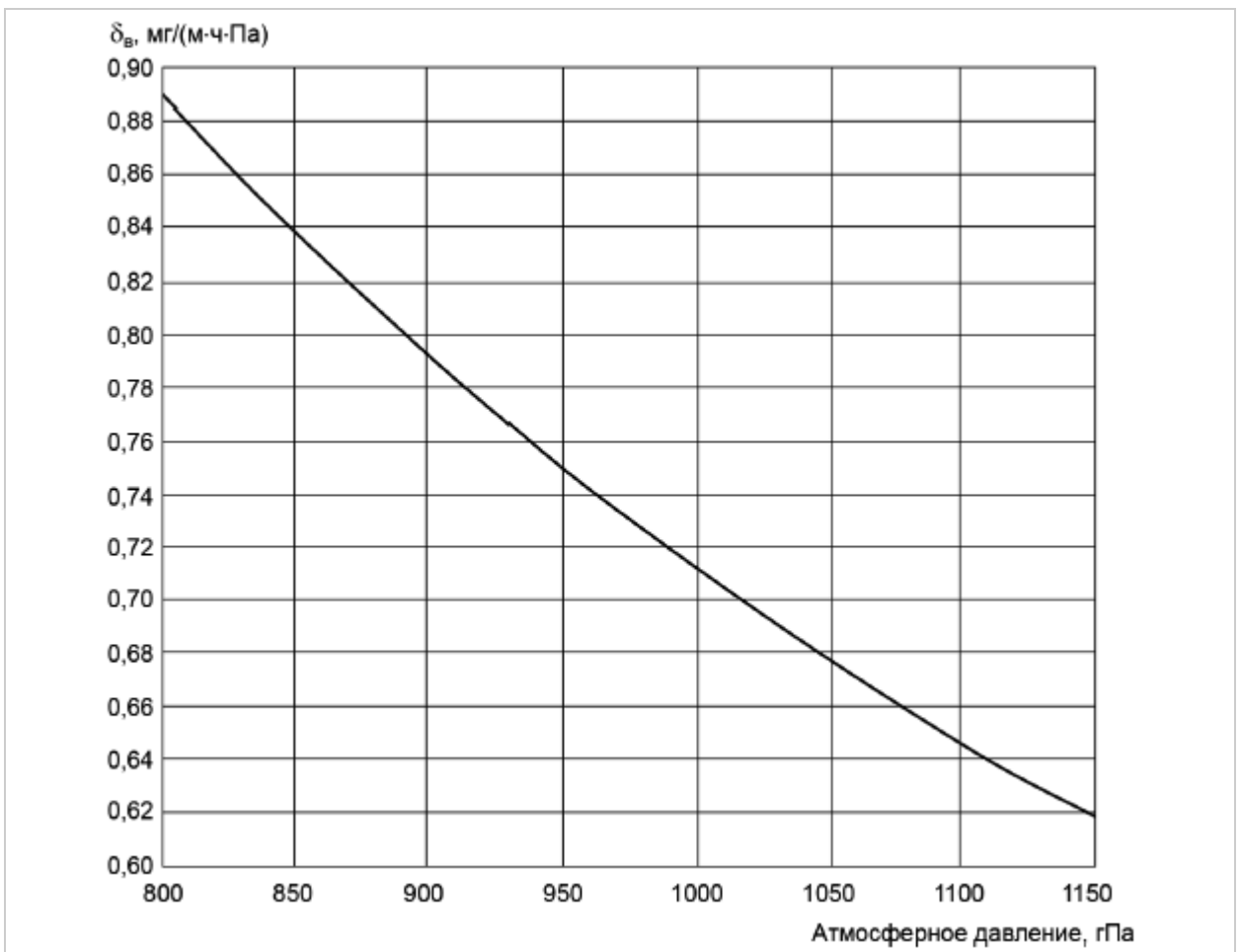
Рисунок Б.1 - Паропроницаемость воздуха при температуре 23°C
