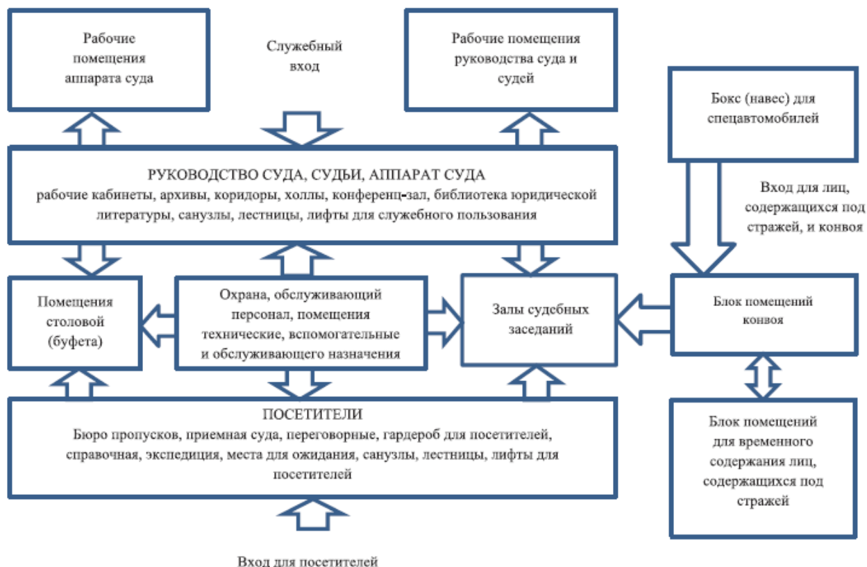
Рисунок 6.1 - Схема функциональной взаимосвязи основных групп помещений зданий судов (для арбитражных судов без блока помещений для конвоя и лиц содержащихся под стражей)". Пункт 6.4. Исключить слова: "и может предусматривать подъем пола".
