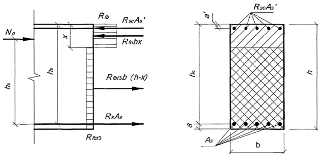
Рисунок 11 - Схема усилий и эпюра напряжений в сечении, нормальном к продольной оси изгибаемого предварительно напряженного элемента при его расчете по прочности в стадии обжатия
