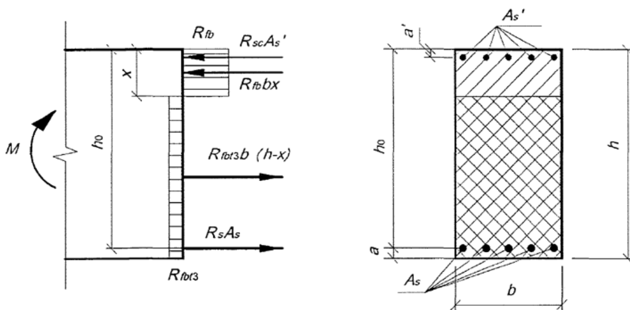
Рисунок 3 - Схема усилий и эпюра напряжений в сечении, нормальном к продольной оси изгибаемого фибробетонного элемента прямоугольного сечения с арматурой, при его расчете по прочности
