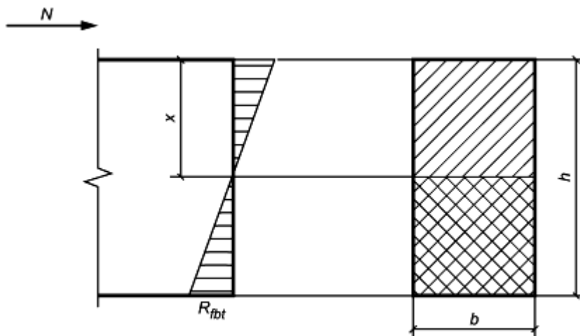
Рисунок 5б* - Схема усилий и эпюра напряжений в сечении, нормальном к продольной оси внецентренно сжатого фибробетонного элемента, рассчитываемого по прочности с учетом сопротивления фибробетона растянутой зоны
