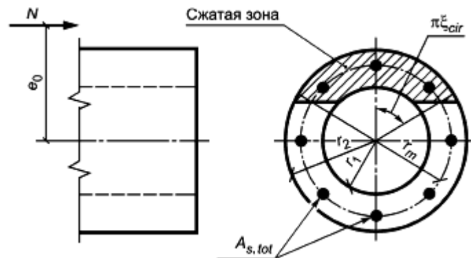
Рисунок 6а* - Схема, принимаемая при расчете кольцевого сечения сжатого элемента
