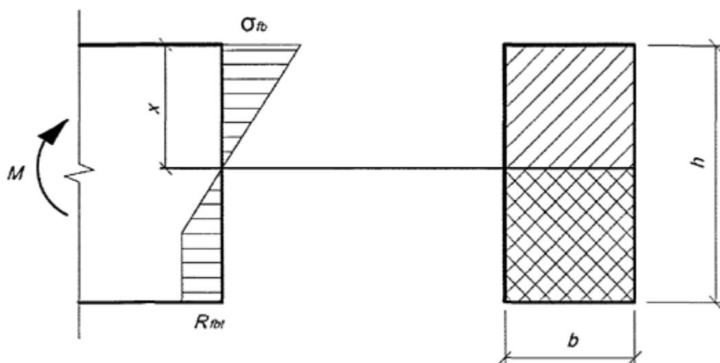
Рисунок 2 - Схема усилий и эпюра напряжений в сечении, нормальном к продольной оси изгибаемого фибробетонного элемента прямоугольного сечения без арматуры при его расчете по прочности
