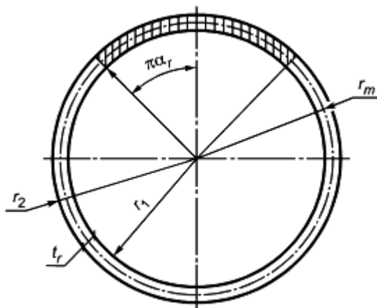
Рисунок 5а* - Схема кольцевого сечения фибробетонного элемента, принимаемая при его расчете по прочности на изгиб
