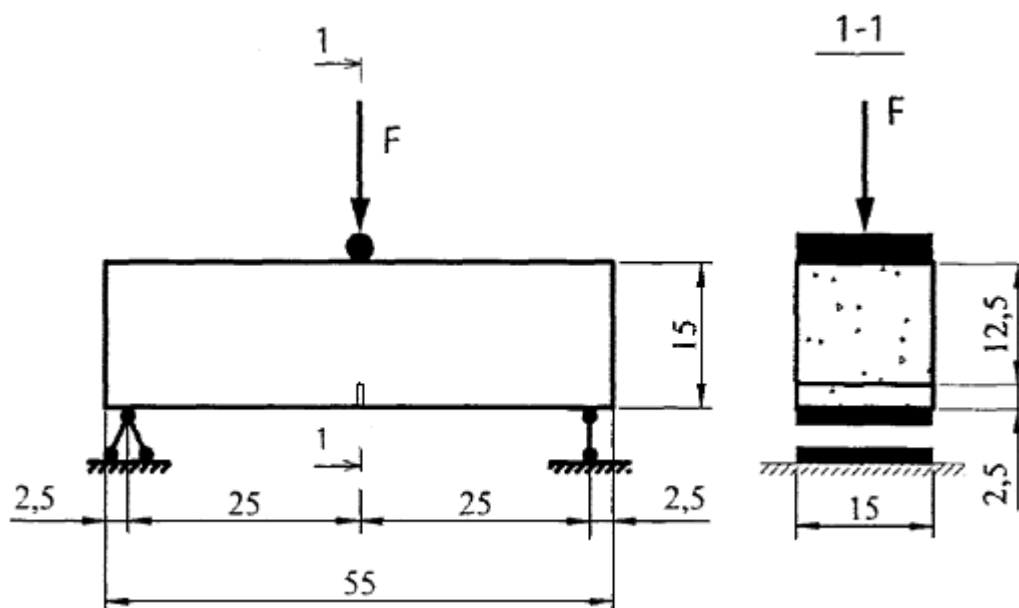
Рисунок Б.1 - Схема испытания образца
