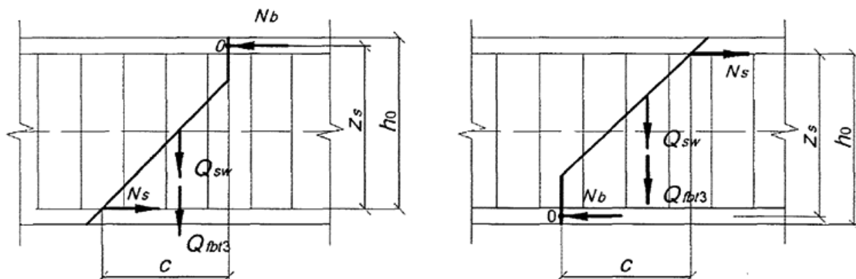
Рисунок 7 - Схема усилий при расчете элементов по наклонному сечению на действие моментов
