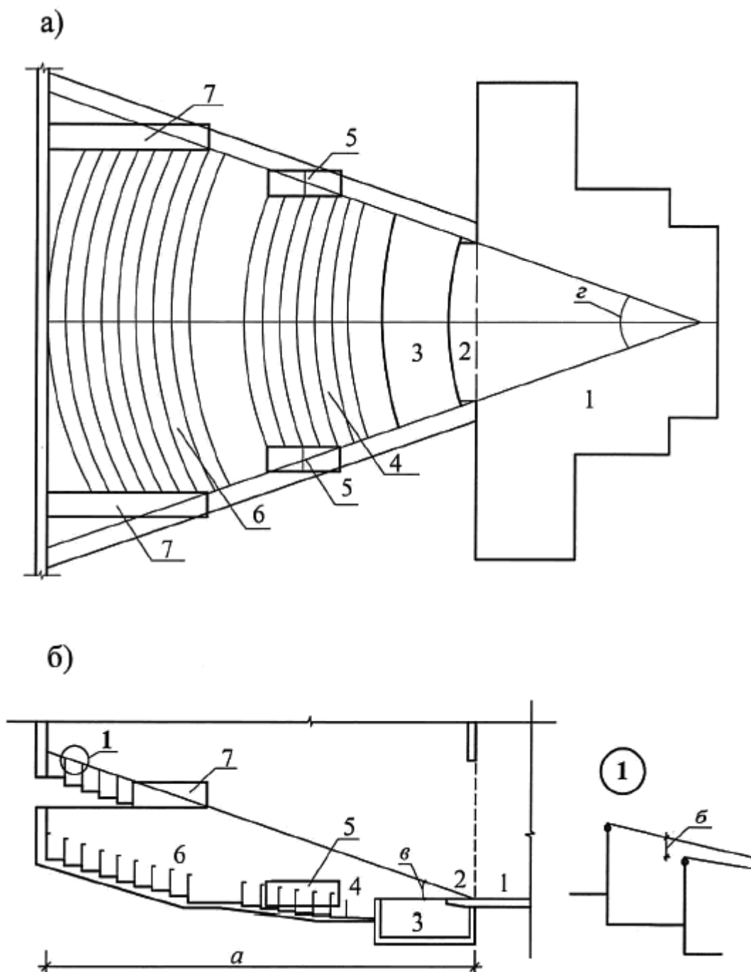
а - план, б - разрез; 1 - сцена; 2 - авансцена; 3 - оркестровая яма; 4 - партер; 5 - ложи; 6 - амфитеатр; 7 - балконы а - длина зала, б - превышение луча зрения зрителя над головой впереди сидящего - см. таблицу Б.1 (приложение Б); в - вертикальный угол размещения зрительских мест, з - горизонтальный угол размещения зрительских мест - см. таблицу Б.2 (приложение Б) Рисунок Б.1 - Схема зрительного зала с колосниковой глубинной порталной сценой Таблица Б.3 - Расчетные параметры зрительного зала
