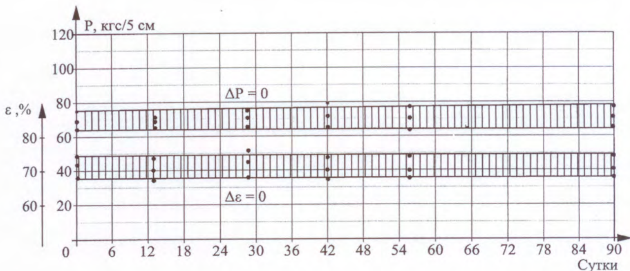
Рис. 1. Изменение прочности (1) и относительного удлинения (2) образцов рулонного материала "Техноласт-Барьер" при воздействии 15-% раствора NaOH
