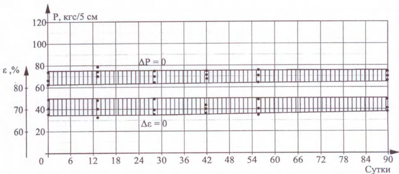
Рис. 2. Изменение прочности (1) и относительного удлинения (2) образцов рулонного материала "Техноласт-Барьер" при воздействии 15-% раствора H_2SO_4
