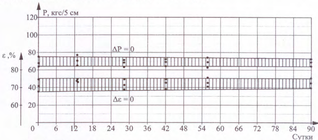
Рис. 3. Изменение прочности (1) и относительного удлинения (2) образцов материала "Техноэласт-Барьер" при воздействии насыщенного раствора NaCl
