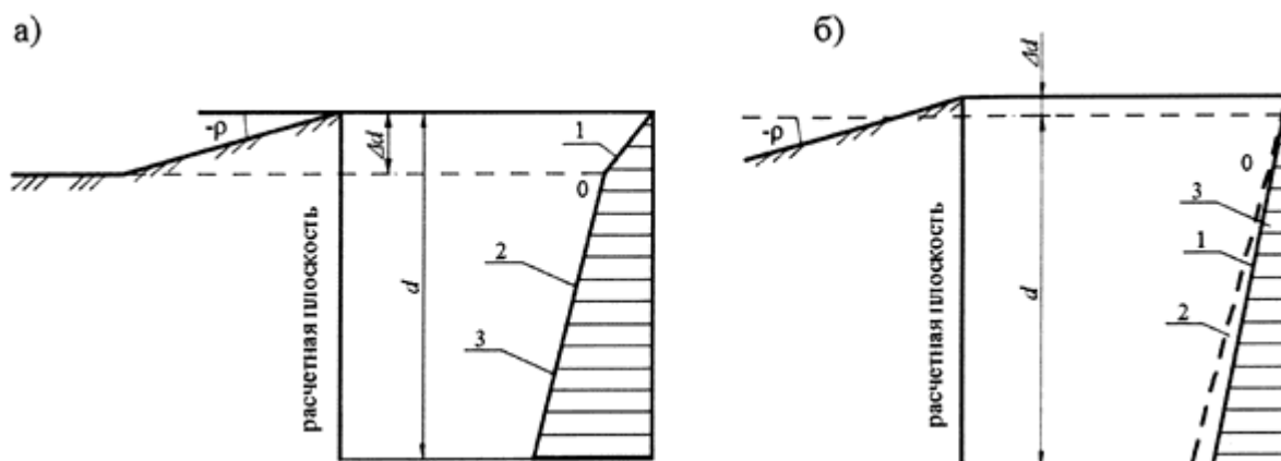
1, 2, 3 - эпюры
