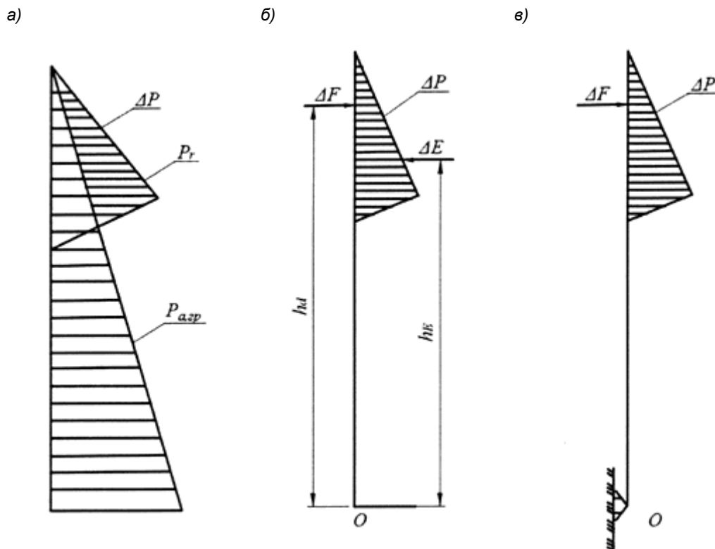
Рисунок Е.3 - Эпюра превышения реактивного давления грунта над активным (а), схема к определению нагрузки \Delta F (б) и расчетная схема (в)
