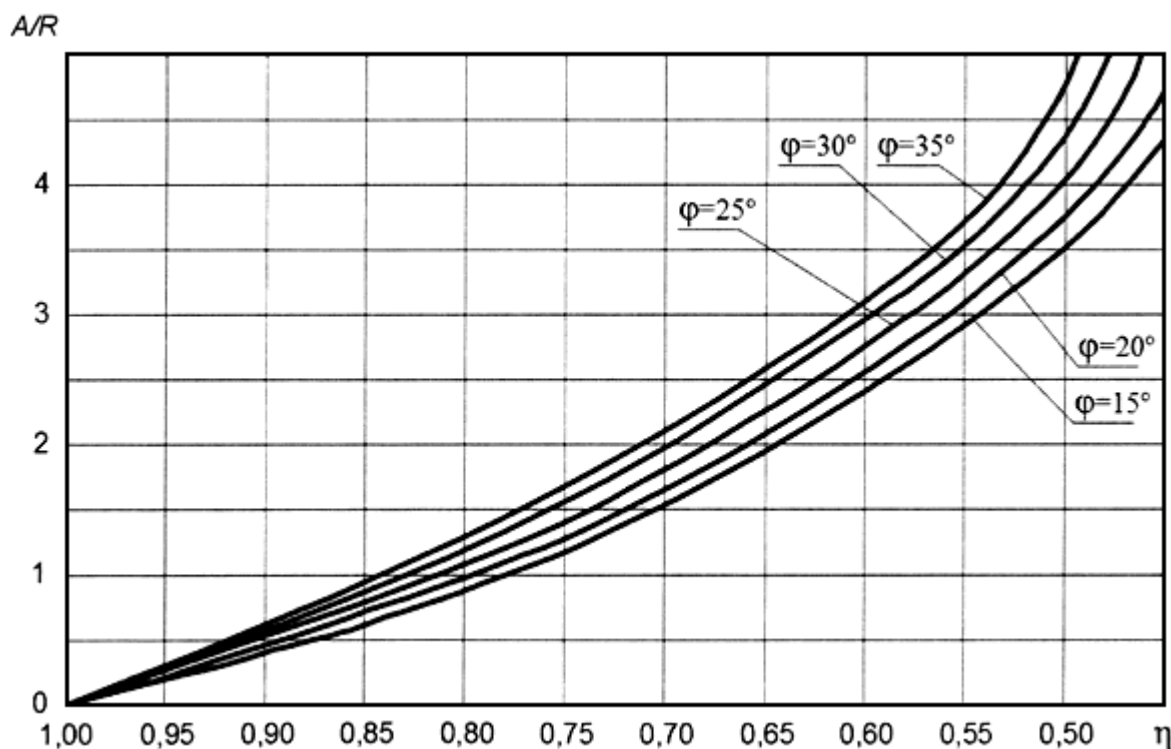
Рисунок 14.2 - График изменения коэффициента \eta
