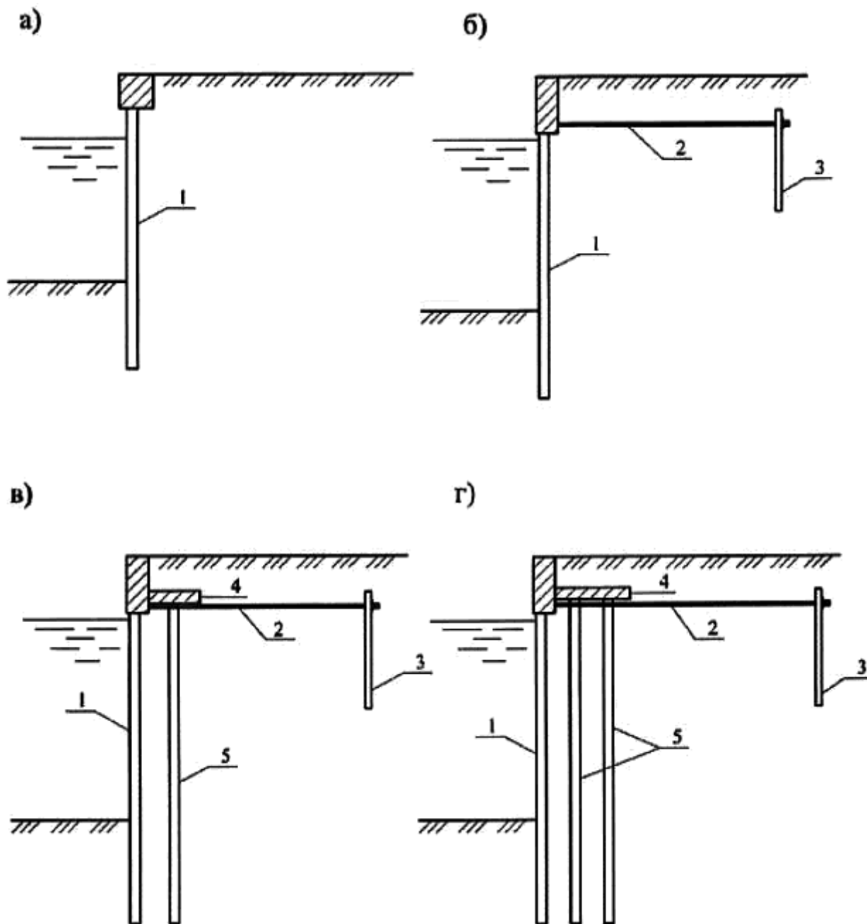
а) - незаанкеренный (безанкерный) больверк; б) - заанкеренный больверк с одним ярусом анкеров; в) - заанкеренный больверк с экранирующей стенкой; г) - заанкеренный больверк с двумя экранирующими стенками; 1 - лицевая шпунтовая стенка; 2 - анкерная тяга; 3 - анкерная опора; 4 - разгрузочная платформа (плита); 5 - экранирующая стенка
