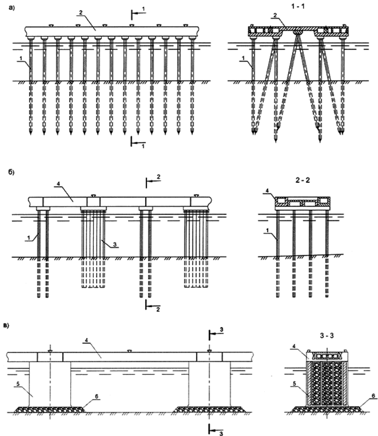
Рисунок 5.2 - Причалные сооружения сквозного типа
