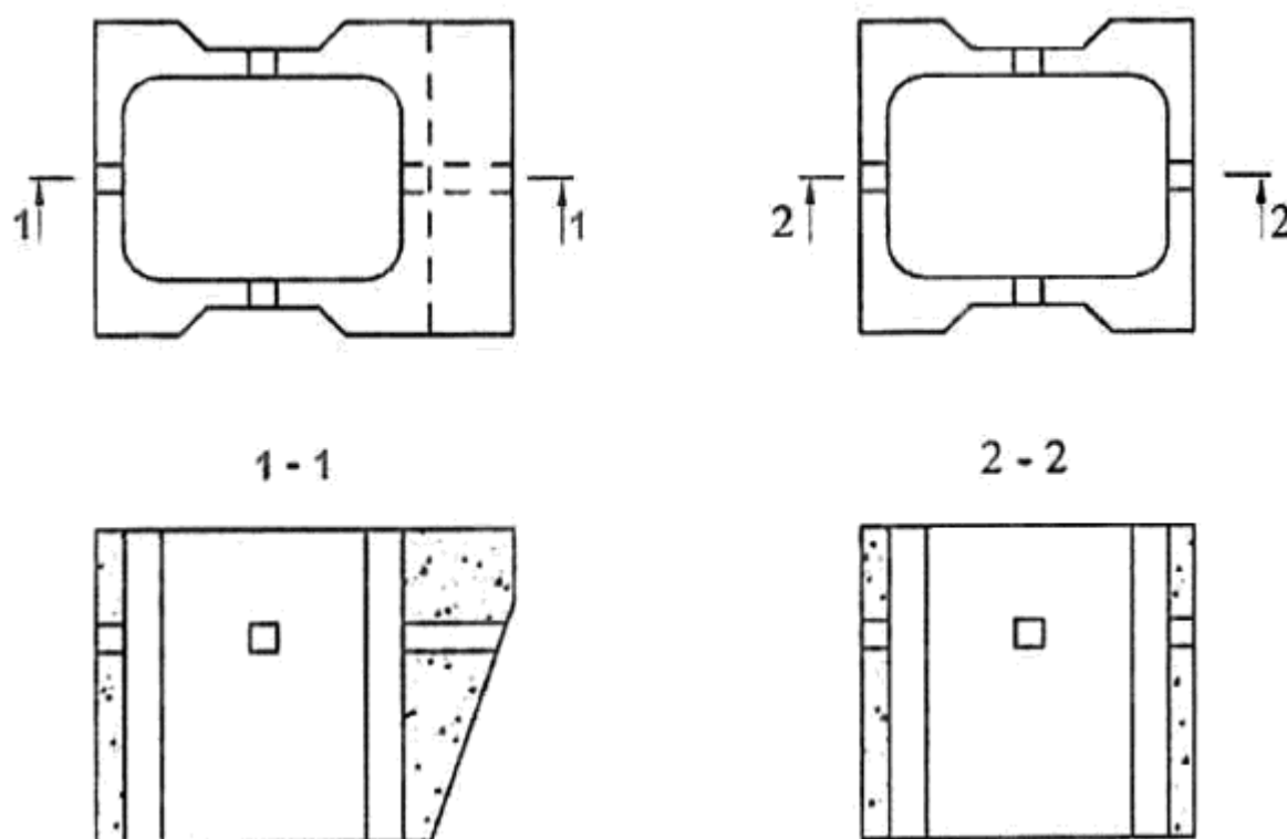
Рисунок 10.1 - Типы пустотелых массивов
