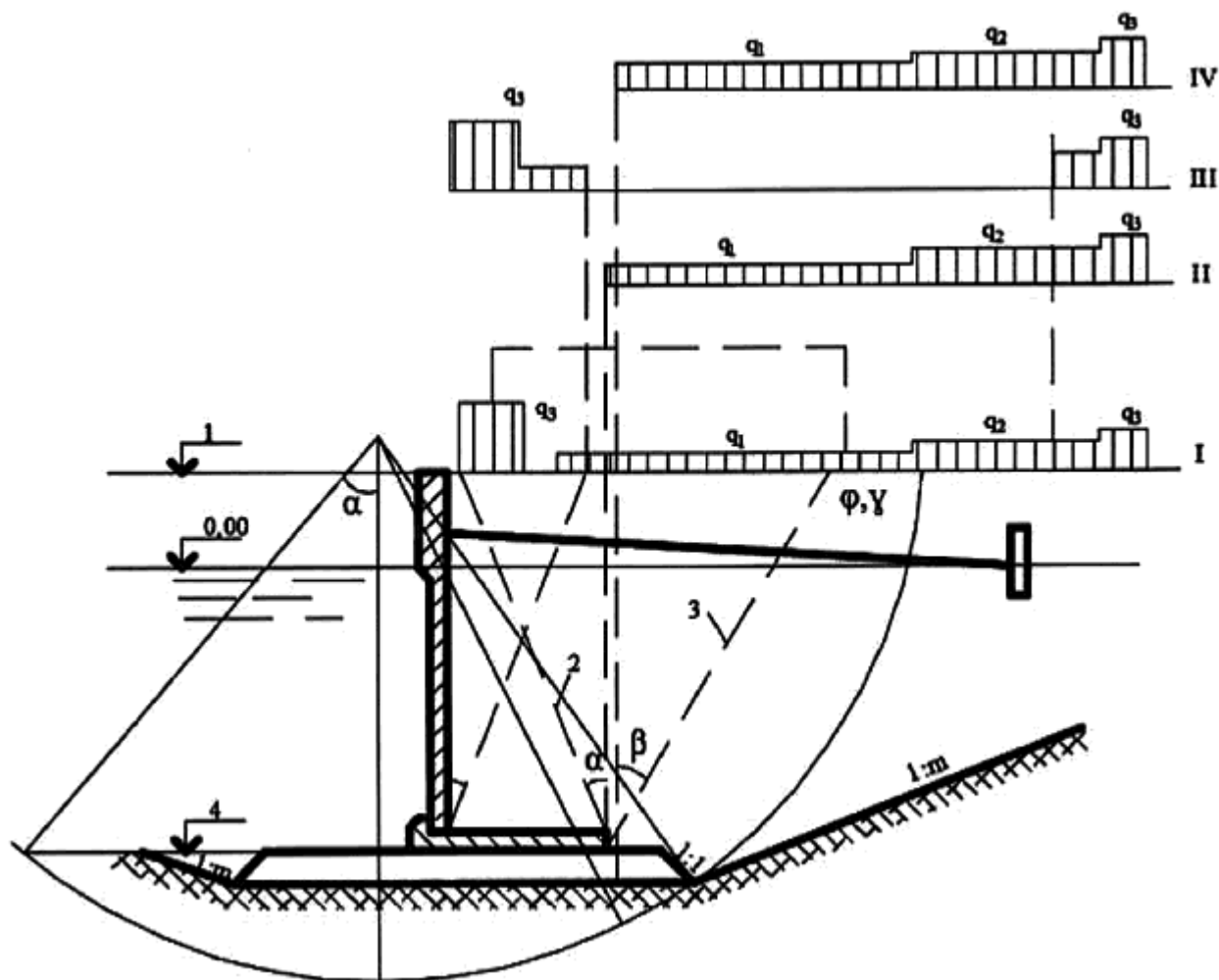
1 - отметка кордона; 2 - плоскость восприятия распора; 3 - плоскость обрушения; 4 - отметка дна; I-IV - схемы нагружения
