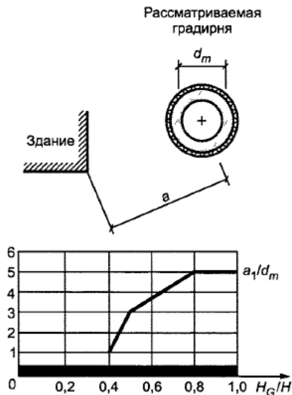
Рисунок Д.4 - Помехи "градирня-здание" в зависимости от отношения H_G/H и верхнего предела
