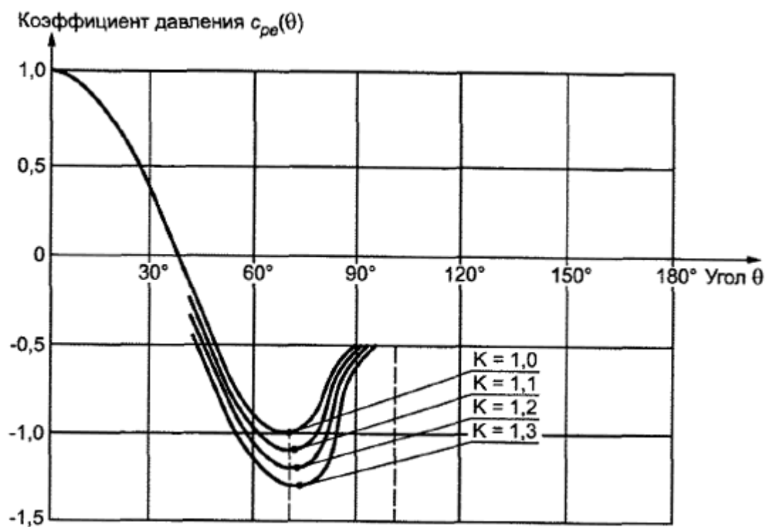
Рисунок Д.1 - Значение коэффициентов внешнего давления c_{pe}(\theta) в зависимости от угла \theta и коэффициентов К 1.0 - К 1.3
