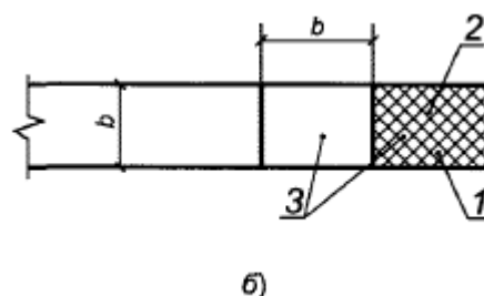
б - при местной краевой нагрузке по всей ширине элемента;
