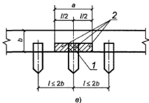
в, г - при местной нагрузке в местах опирания концов прогонов и балок;
