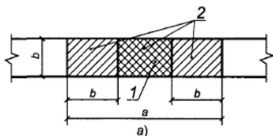
а - при местной нагрузке по всей ширине элемента;
