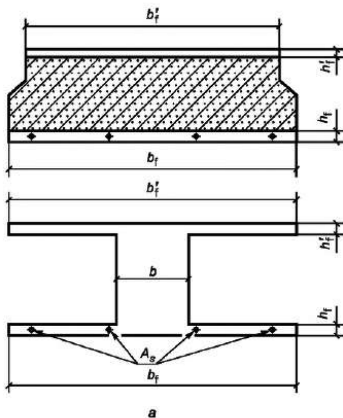
а - плита перекрытия трехслойная;
