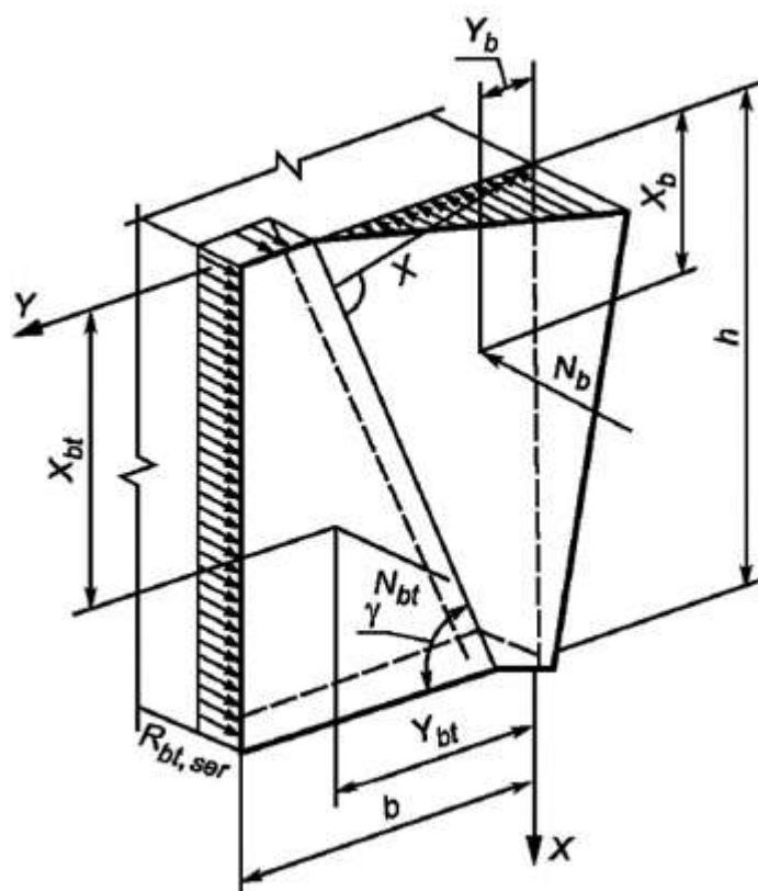
Рисунок Г.3 - Напряженно-деформированное состояние в поперечном сечении элемента со сжатой зоной в форме "удлиненной" трапеции (случай В)
