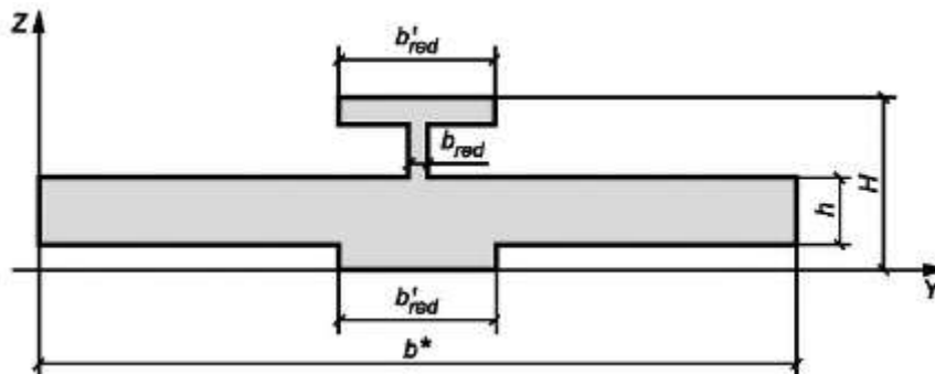
Рисунок 7.21 - Приведенное поперечное сечение ограждающих конструкций
