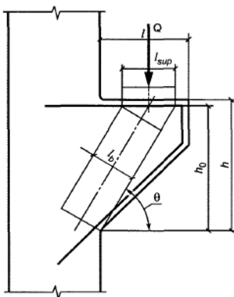
Рисунок 7.10 - Схема для расчета коротких консолей
