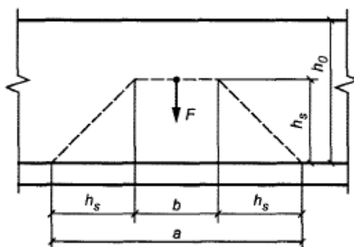
Рисунок 7.16 - Схема для расчета железобетонных элементов на отрыв
