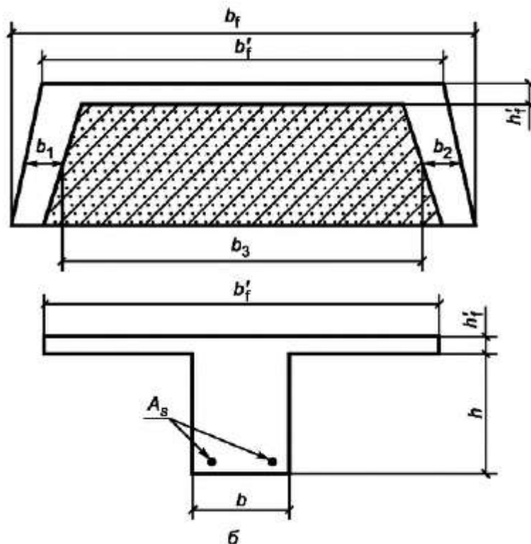
б - плита перекрытия с боковыми несущими гранями
