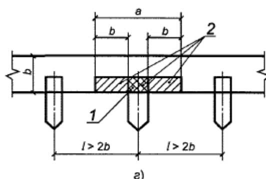
в, г - при местной нагрузке в местах опирания концов прогонов и балок;
