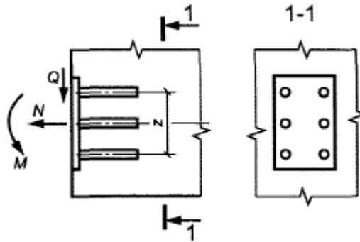
Рисунок 7.17 - Схема усилий, действующих на закладную деталь
