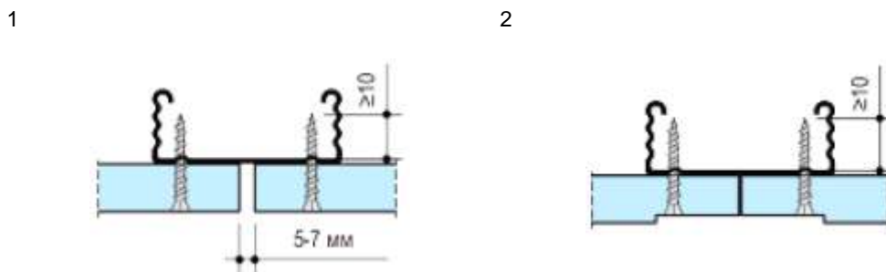
1 - с прямой кромкой; 2 - фальцевой кромкой
