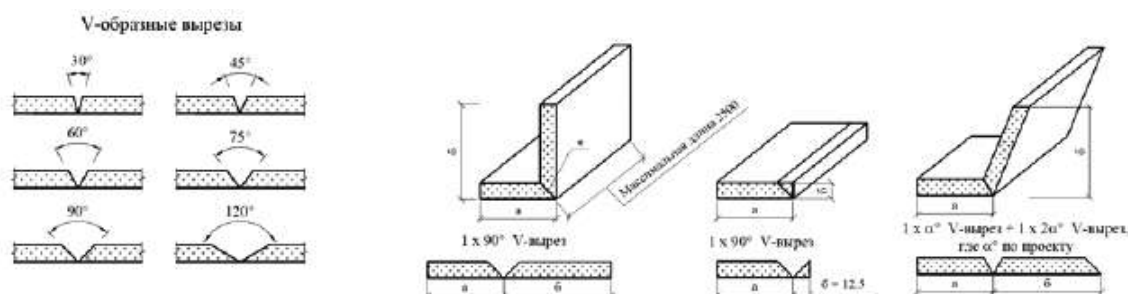
Угловые элементы конструкций ( a + b \leq 500 мм)
