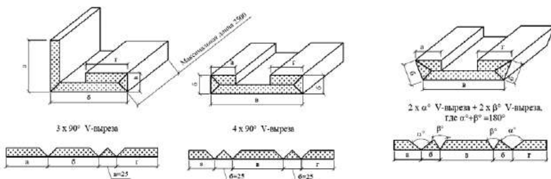
П-образные элементы конструкций ( a + b + c + d \leq 500 мм)
