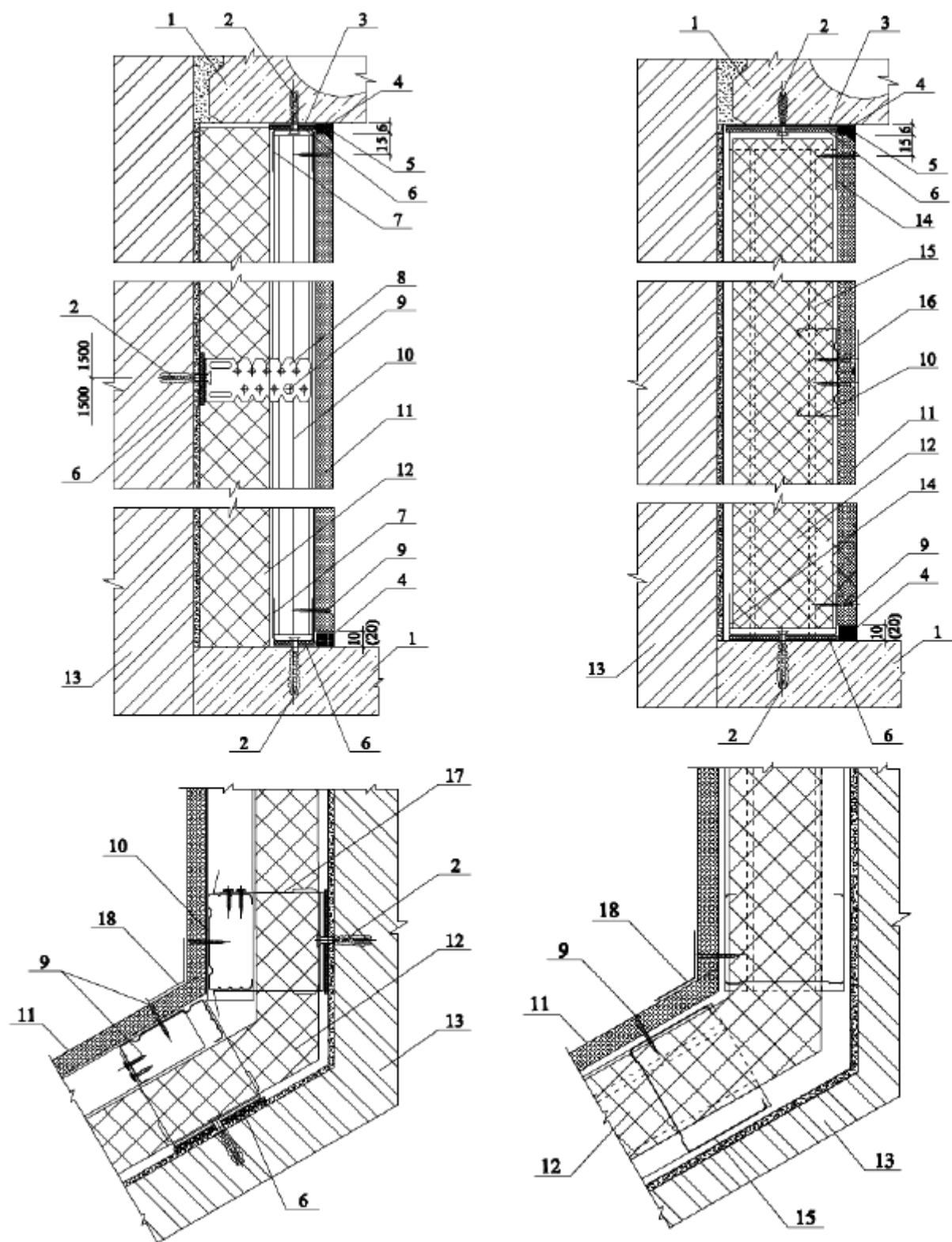
а - на прямых подвесах; б - на отnose
