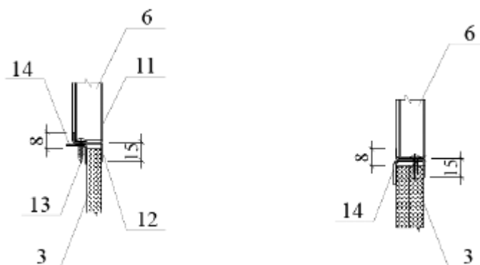
а - вертикальный разрез; б - горизонтальный разрез
