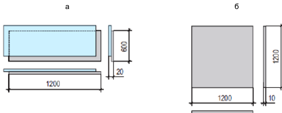
а - элемент пола; б - влагостойкий гипсоволокнистый лист ГВЛВ
