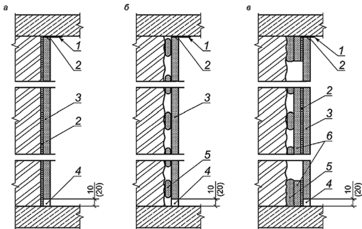
а - крепление гипсокартонных листов или гипсовых плит на ровное основание; б - крепление гипсокартонных листов или гипсовых плит на основание с неровностью до 20 мм; в - крепление гипсокартонных листов или гипсовых плит на основание с неровностью свыше 20 мм; 1 - разделительная лента; 2 - шпаклевка; 3 - лист ГКЛ или ГВЛ или плита ГСП; 4 - герметик; 5 - клей; 6 - полоса ГКЛ или ГВЛ или плита ГСП
