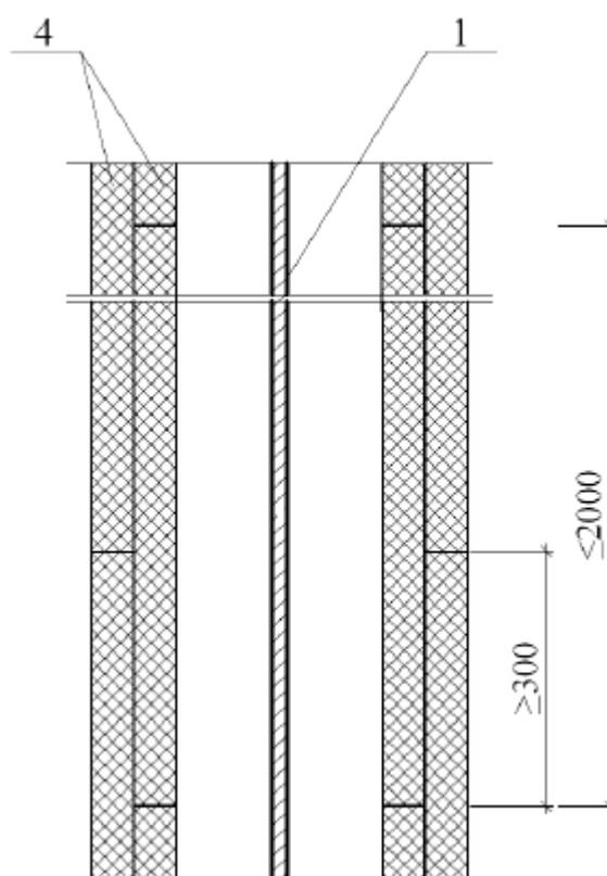
Вертикальный разрез
