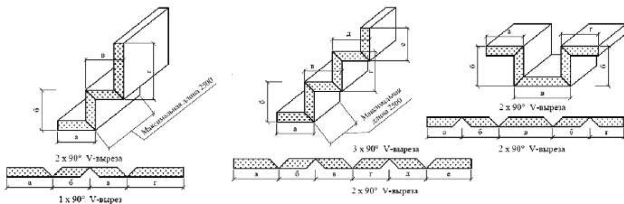
Ступенчатые элементы конструкций (сумма длин участков элемента \leq 500 мм)
