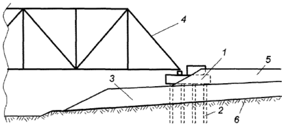
1 - тело устья; 2 - столбы фундамента длиной до 15 м; 3 - уширенная площадка; 4 - пролетное строение; 5 - подходная часть насыпи; 6 - естественная поверхность грунта
