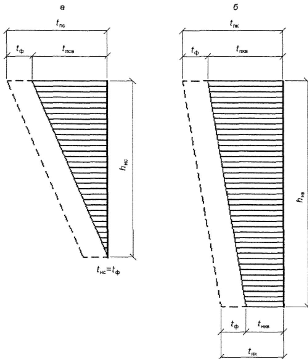
а - сквозная термоопора; б - коаксиальная термоопора
