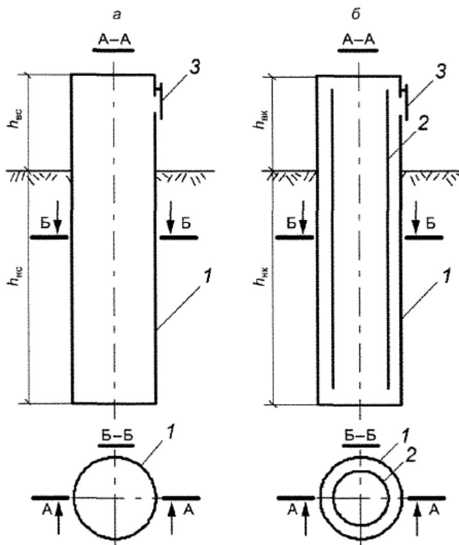
а - сквозная термоопора; б - коаксиальная термоопора
