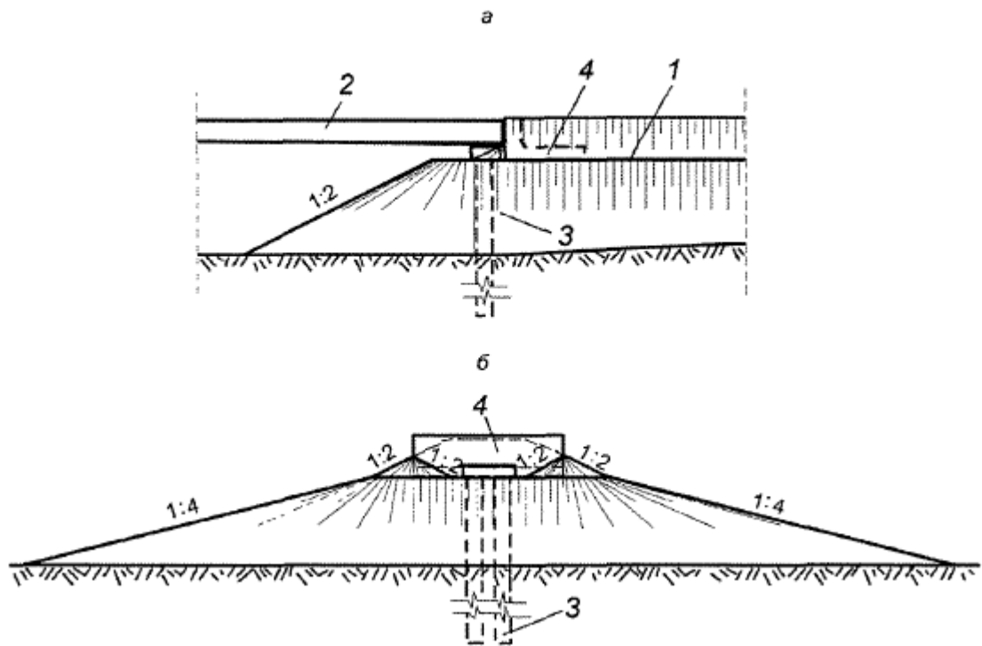
а - фасад оси моста со стороны пролета; б - вид вдоль оси моста со стороны пролета 1 - подходная часть насыпи; 2 - пролетное строение; 3 - безростверковая опора, воспринимающая нагрузку от пролетного строения; 4 - стенка с горизонтальной плитой, воспринимающая нагрузку со стороны насыпи
