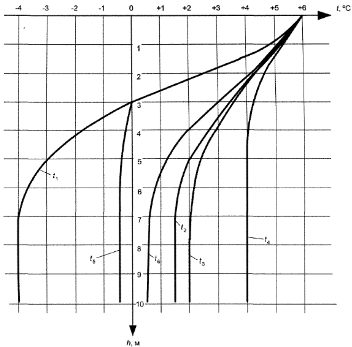
Рисунок К.7 - Распределение температуры t грунта по глубине h для изолированных зон 1-6 на рисунке К.6 на момент окончания теплого периода года (данные для примера расчета) Таблица К.4 - Расчет температуры грунта в точке О на глубине 3,0 м на момент окончания теплого периода года (рисунок К.6)
