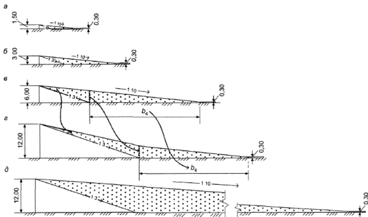
а, б, в, г - для насыпей с высотой 1,5; 3,0; 6,0; 12,0 м соответственно, расположенных в условиях равнины; д - для насыпи высотой 12,0 м, расположенной в логе
