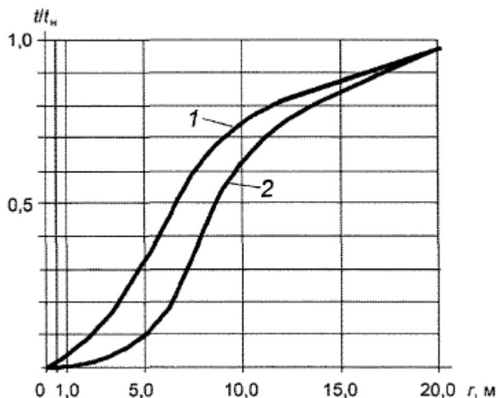
Рисунок И.2 - "Растекаемость" намерзших локальных массивов за теплый период года - отношение температуры t на начало холодного периода к температуре t_n на начало теплого периода года при фоновой температуре минус 0^{\circ}\text{C} (кривая 1) и плюс 0^{\circ}\text{C} (кривая 2)
