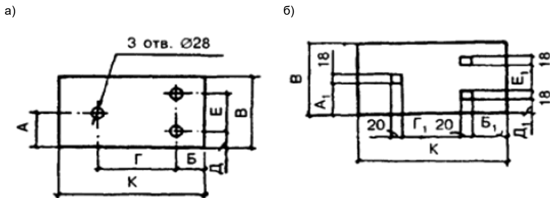
Рисунок 1 - Крепление рельса к полушпалам с помощью шурупов (а) и с помощью костылей (б) Таблица 1 - Размеры подкладок скреплений
