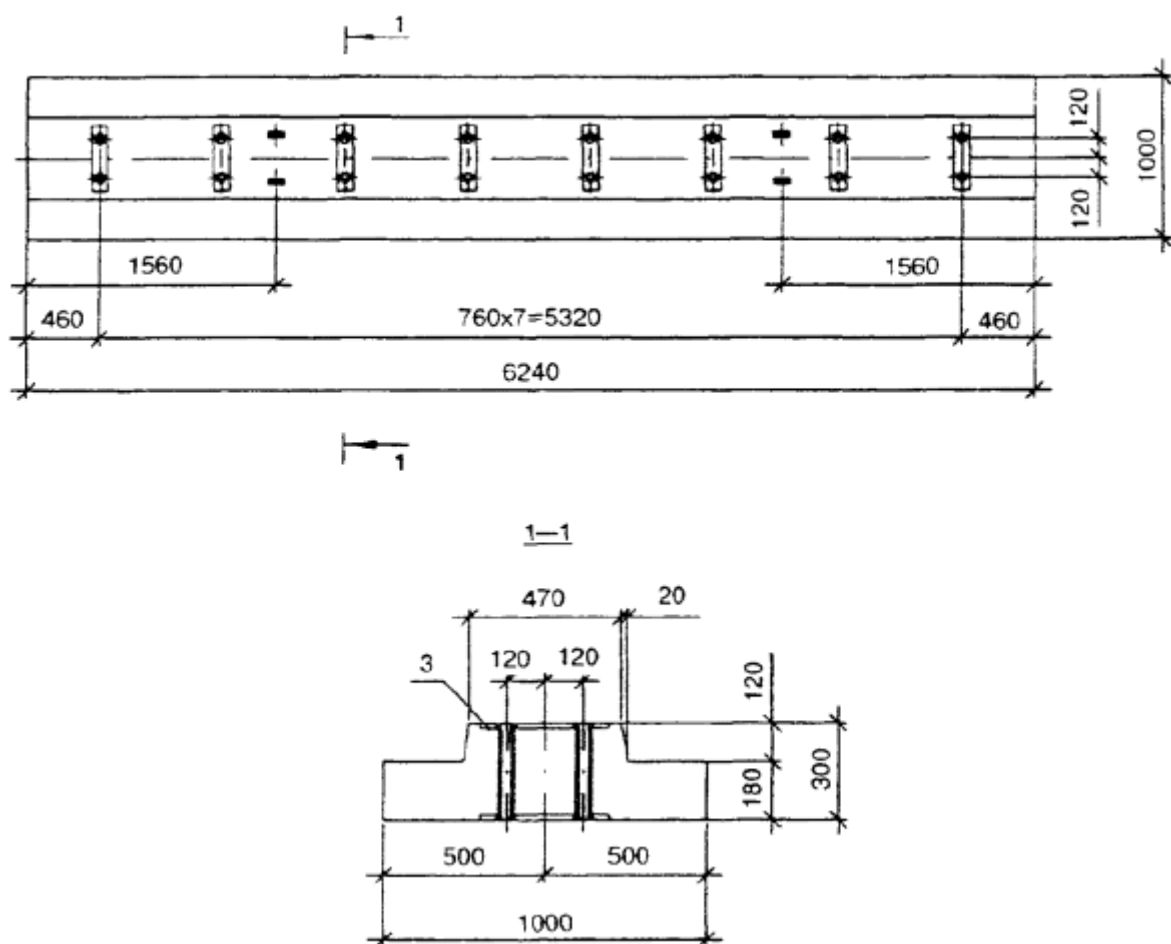
Рисунок Д.6 - Железобетонная балка типа БРК-6.24-04
