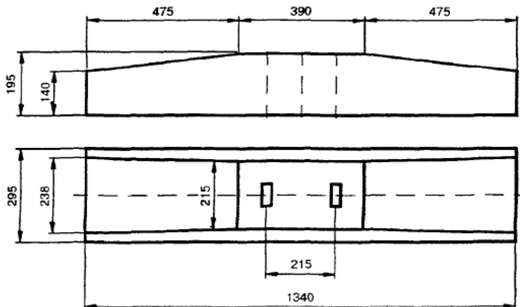
Рисунок Д.3 - Железобетонная полушпала типа ПШН4-13-325-1 Б3
