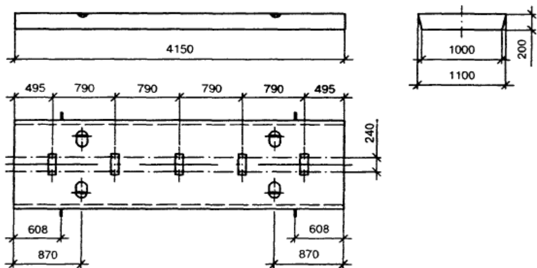
Рисунок Д.5 - Железобетонная плита
