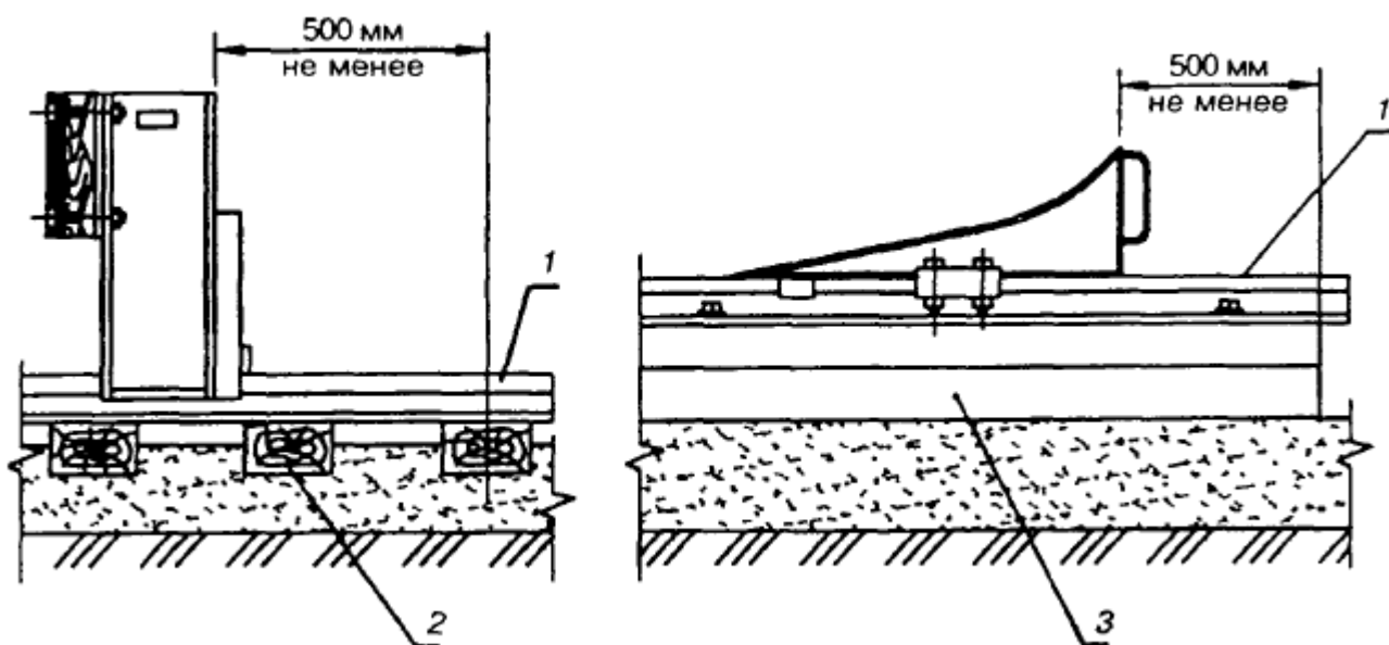
г) установка тупиковых упоров на рельсовой нити
