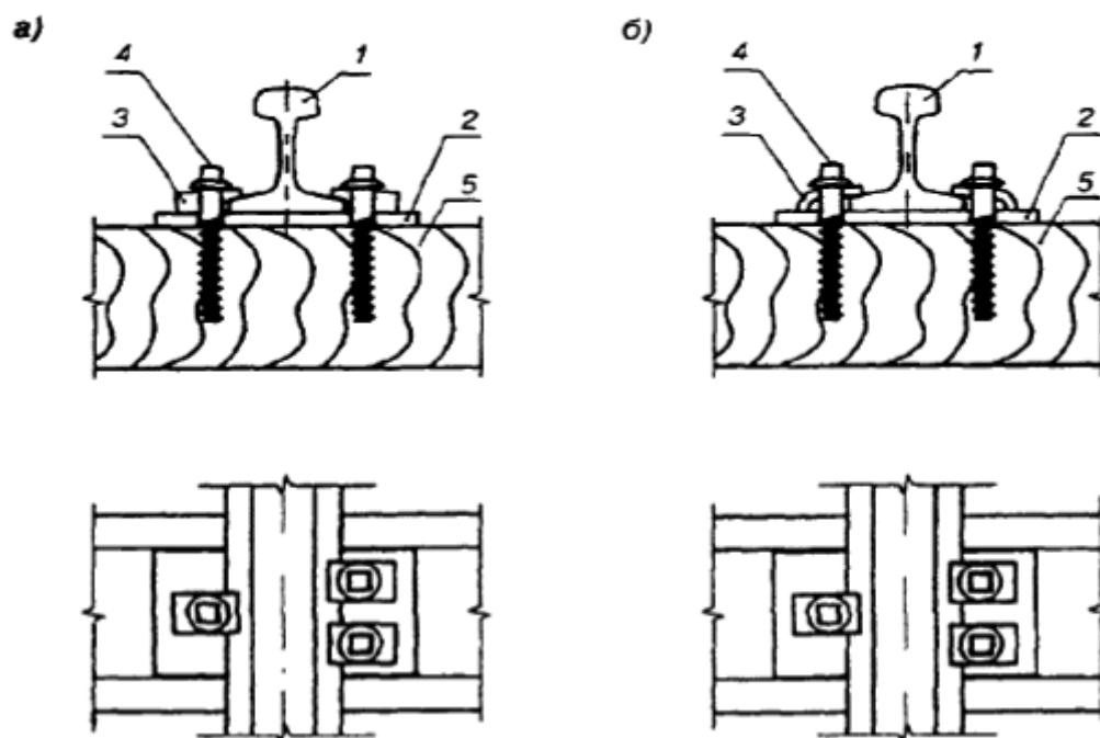
а) - "нормальные" прижимы; б) - "облегченные" прижимы 1 - рельс; 2 - подкладка; 3 - прижим; 4 - путевой шуруп; 5 - полушпала
