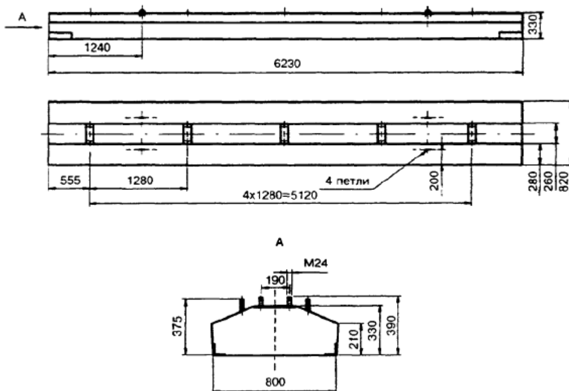
Рисунок Д.4 - Железобетонная балка типа БРП-62.8.3
