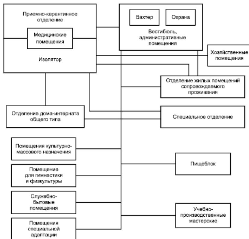
Рисунок А.2 - Схема взаимосвязей жилых групп и помещений дома-интерната для граждан, имеющих психические расстройства, специального дома-интерната и отделений жилых помещений сопровождаемого проживания Приложение Б
