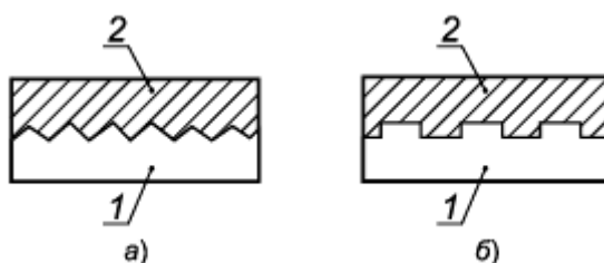
а - треугольные; б - прямоугольные; 1 - сборный элемент; 2 - монолитный бетон
