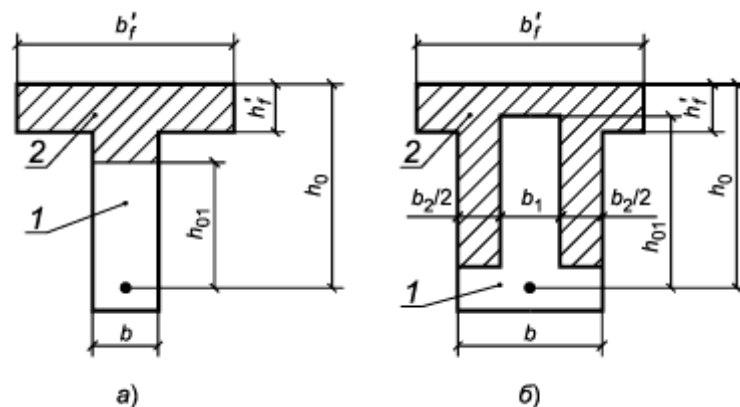
а - тип 1; б - тип 2; 1 - сборный элемент; 2 - монолитный бетон
