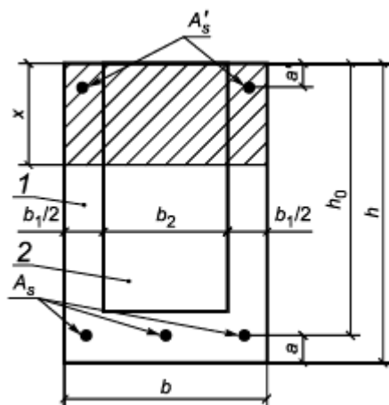
1 - П-образный сборный элемент; 2 - монолитный бетон
