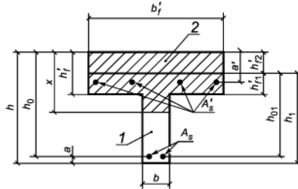
1 - сборный элемент; 2 - монолитный бетон
