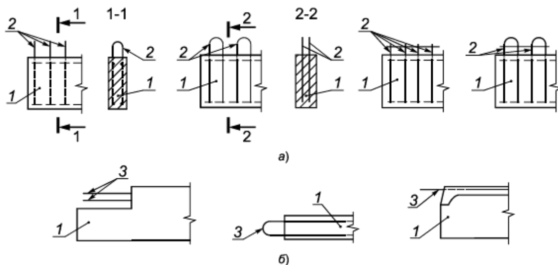
а - поперечная арматура; б - продольная арматура; 1 - сборный элемент; 2 - выпуски поперечной арматуры; 3 - выпуски продольной арматуры
