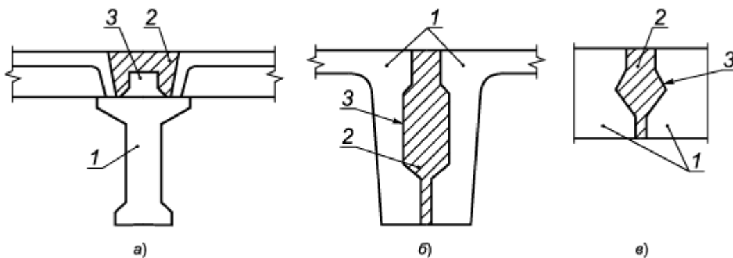
а - ригеля с плитами; б, в - плит между собой; 1 - сборный элемент; 2 - монолитный бетон; 3 - продольный выступ или паз
