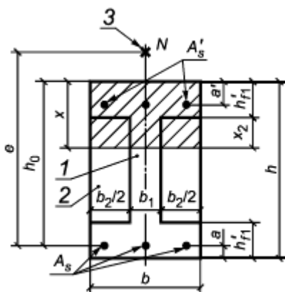
1 - сборный элемент; 2 - монолитный бетон; 3 - точка приложения силы N
