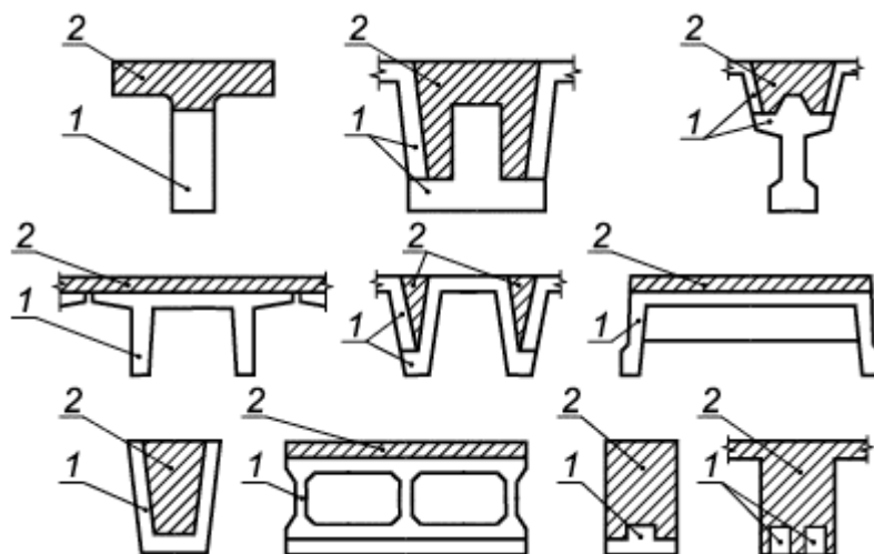
1 - сборный элемент; 2 - бетон омоноличивания
