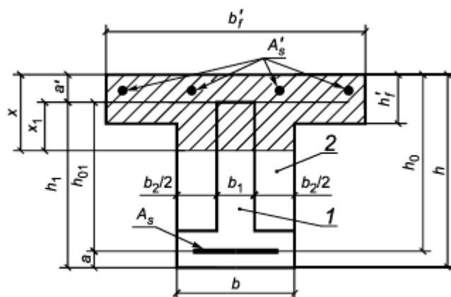
1 - сборный элемент; 2 - монолитный бетон
