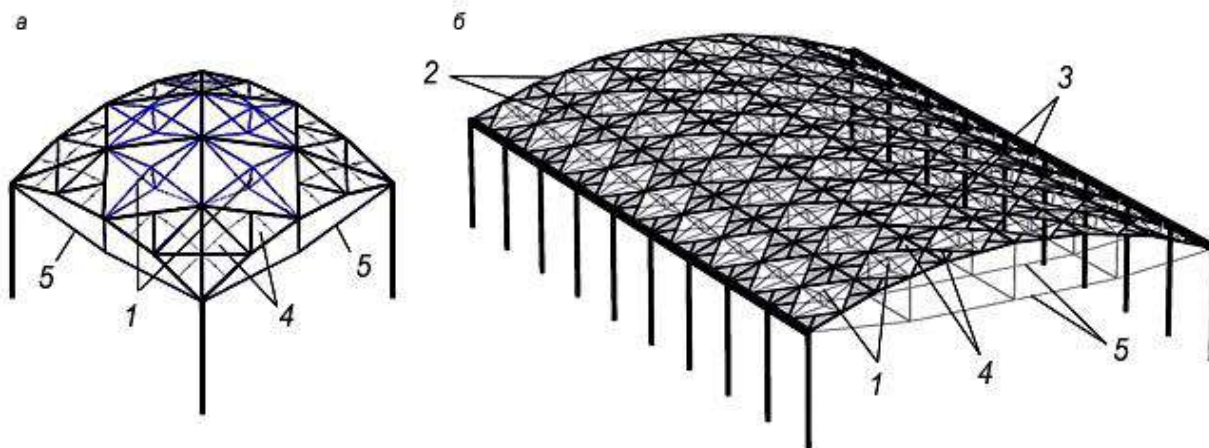
а - оболочка; б - свод с применением линейных элементов; 1 - самоуравновешенная напрягаемая система; 2 - арка; 3 - продольное ребро; 4 - сборные плиты; 5 - затяжка Рисунок 6.7 - Сборные покрытия с большой площадью световых проемов
