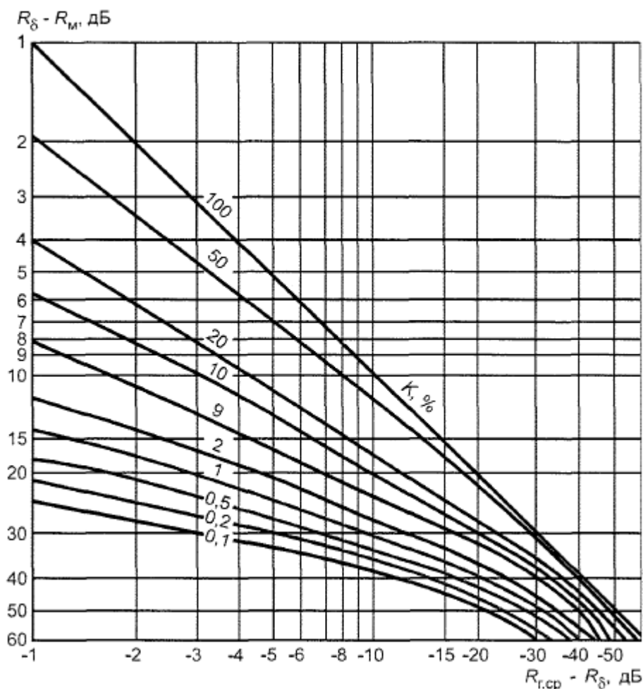
Рисунок 15 - Номограмма для определения средней звукоизоляции неоднородных ограждений
