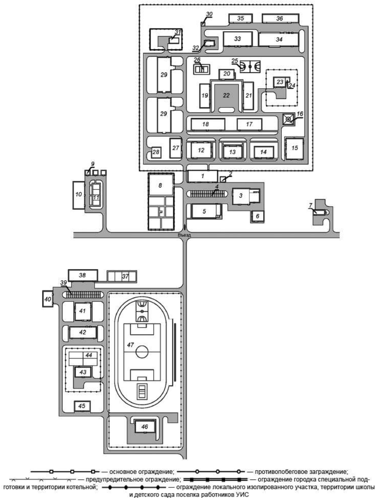
Рисунок В.4 - Схема планировочной организации земельного участка КП (с лимитом наполнения 400 чел.), лист 1
