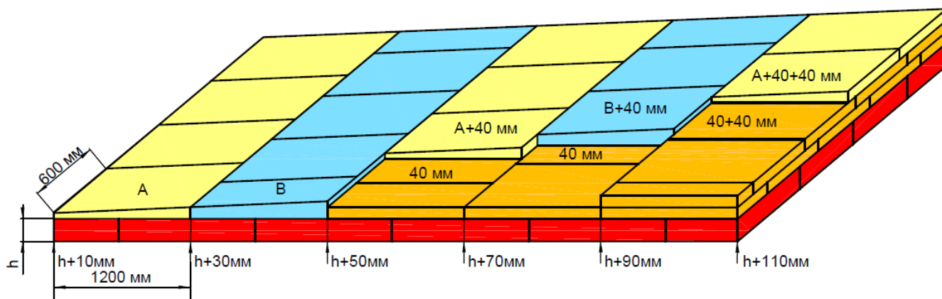
Рис. 5.5. Пример выполнения основного уклона из плит ТЕХНОНИКОЛЬ CARBON PROF SLOPE 1,7%
