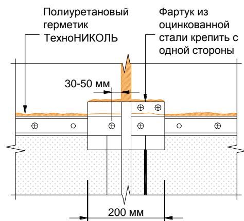
Рис. 5.30 Краевая рейка на стене из бетонных плит
