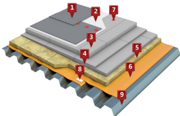
Рис. 4.1. Конструкция системы ТН-КРОВЛЯ Смарт
