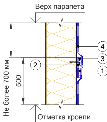
1 – сварной шов; 2 – полоса полимерной мембраны шириной 130 мм; 3 – прижимная рейка ТехноНИКОЛЬ; 4 – кровельный материал на вертикальной поверхности
