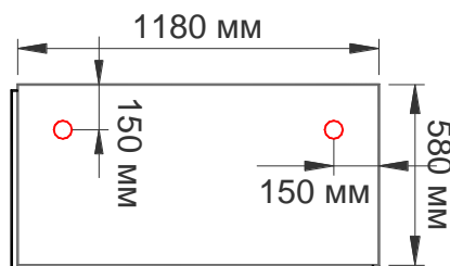
Рис. 5.11. Схема крепления теплоизоляционных плит из экструзионного пенополистирола
