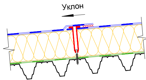
Рис. 5.18 «Встречный» шов
