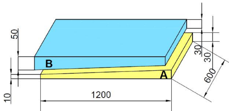
Рис. 5.4. Набор плит клиновидной теплоизоляции ТЕХНОНИКОЛЬ CARBON PROF SLOPE 1,7%
