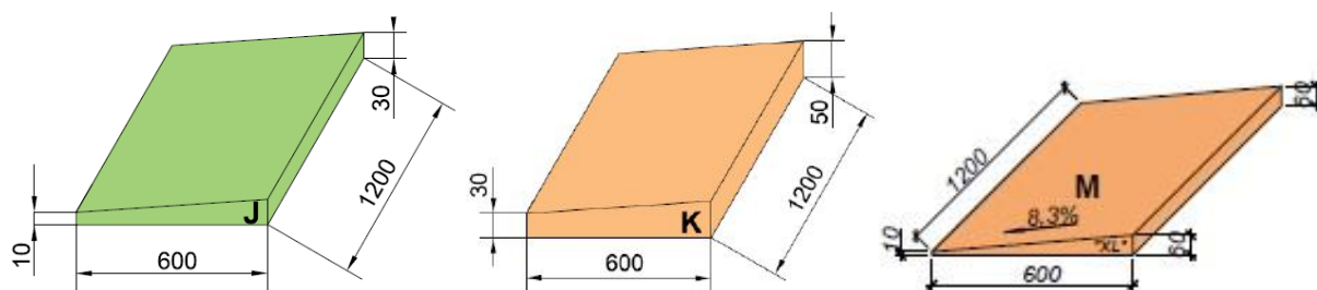
Рис. 5.6. Набор плит ТЕХНОНИКОЛЬ CARBON PROF SLOPE 3,4% и 8,3%
