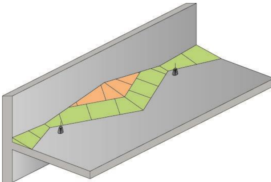
Рис. 5.9 Схема раскладки плит ТЕХНОНИКОЛЬ CARBON PROF SLOPE 3,4% и 8,3 % при устройстве контруклона в парапетной зоне
