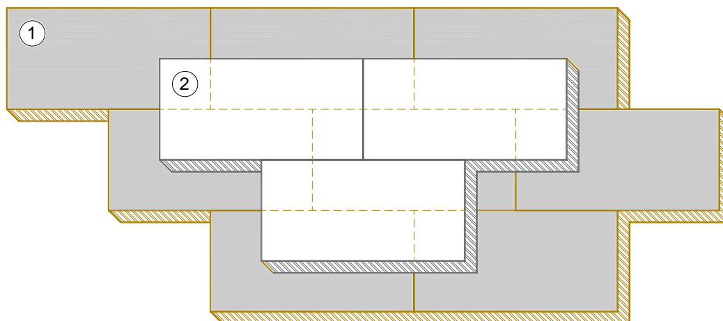
Рис. 5.10 Смещение плит верхнего и нижнего слоев при укладке. 1 – нижний слой плит; 2 – верхний слой плит
