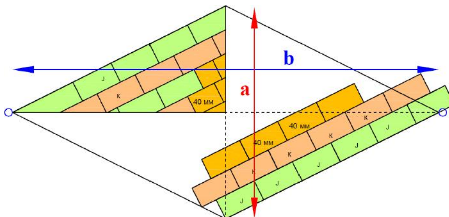
Рис. 5.8. Схема раскладки плит ТЕХНОНИКОЛЬ CARBON PROF 3,4% при создании разуклонки между воронками в ендове
