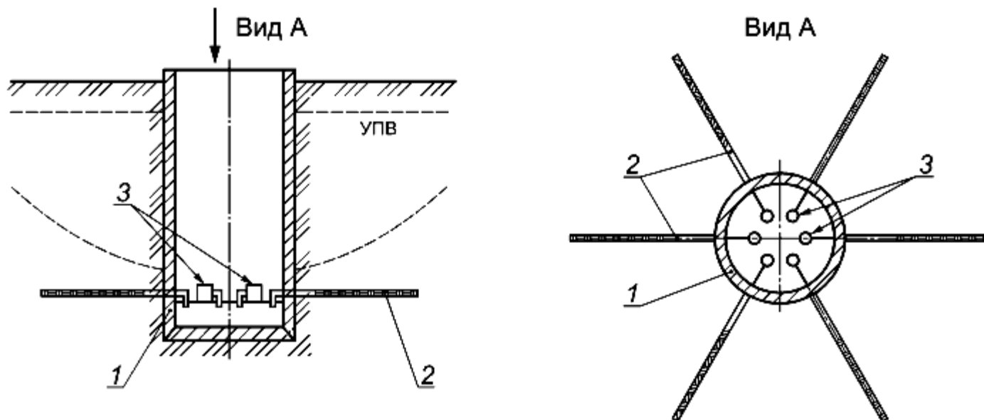
1 - водосборный колодец; 2 - горизонтальные радиальные скважины (дренажи); 3 - насосы Рисунок 7.3* - Лучевой водозабор
