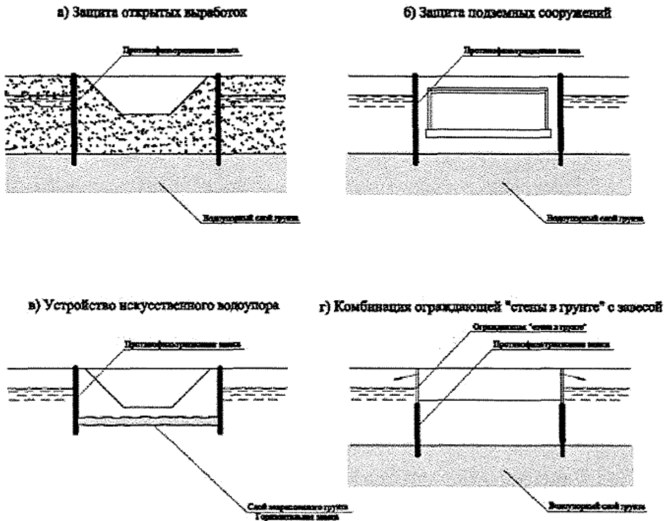
а) - защита открытых выработок; б) - защита подземных сооружений; в) - устройство искусственного водопора; г) - комбинация ограждающей "стены в грунте" с завесой
