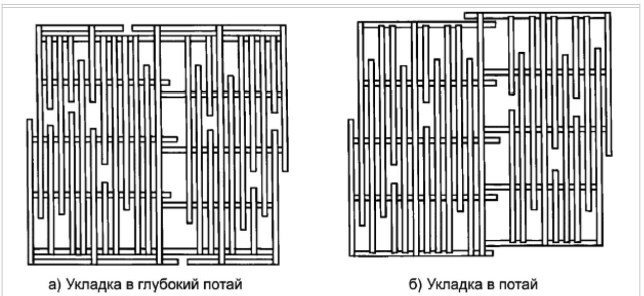
Рисунок А.7 - Способы укладки пиломатериалов разных длин в сушильные пакеты
