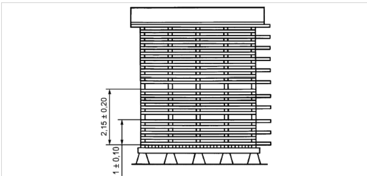
Рисунок А.9 - Горизонтальные каналы в рядовом штабеле
