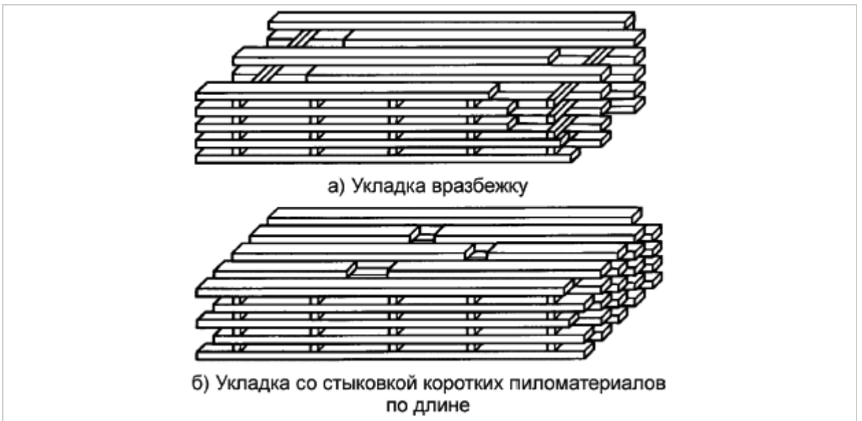
Рисунок А.7 - Способы укладки пиломатериалов разных длин в сушильные пакеты
