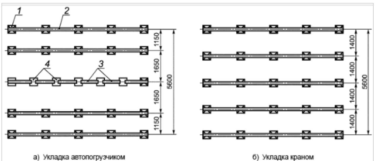
Рисунок А.3 - Планировка групп штабелей при укладке козловым (а) и башенным (б) кранами
