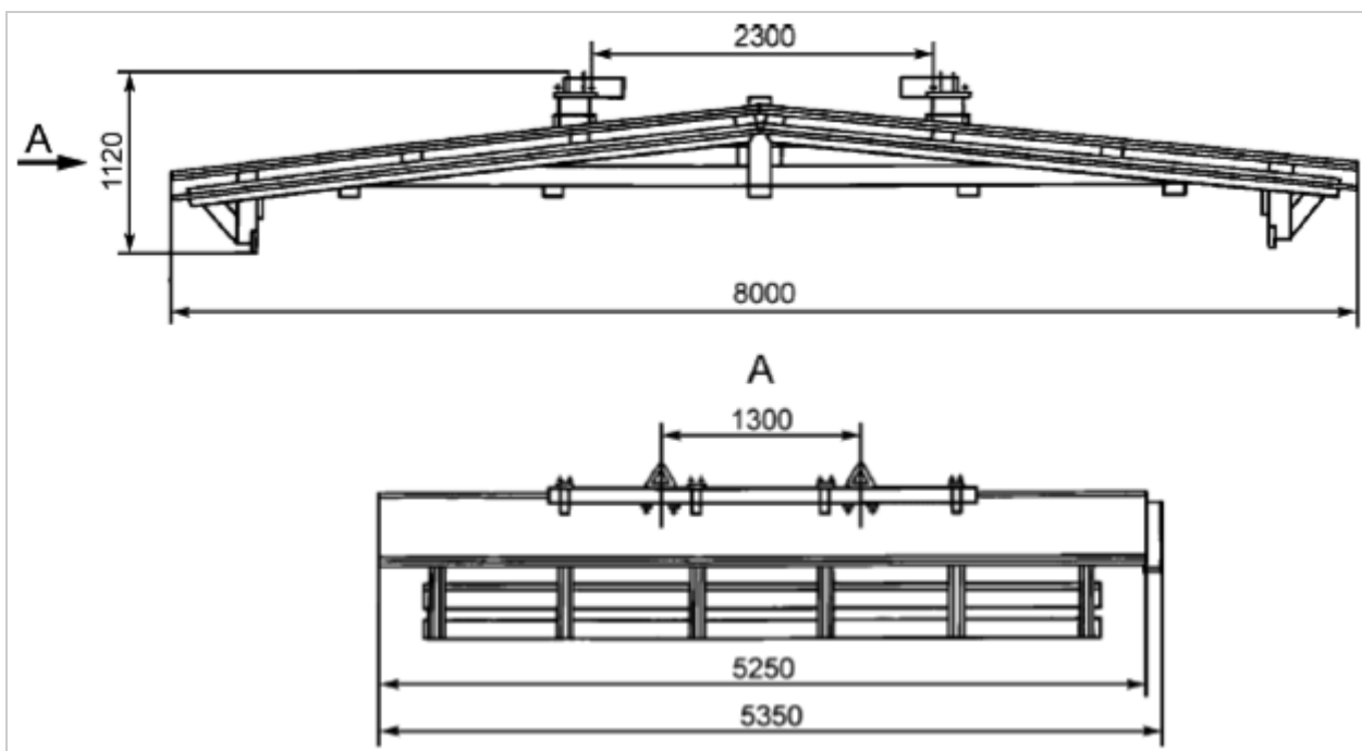
Рисунок Г.1 - Съёмная крыша, применяемая при формировании штабелей краном
