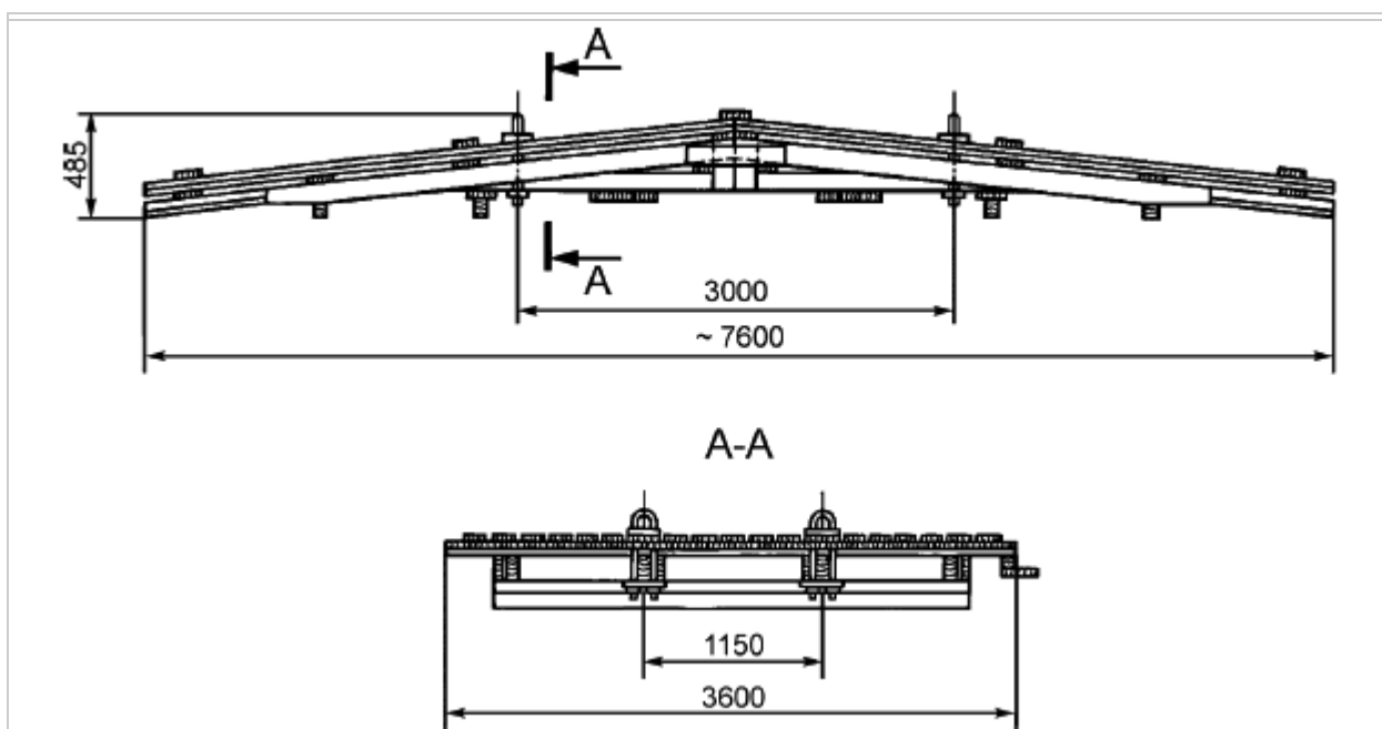
Рисунок Г.1 - Съёмная крыша, применяемая при формировании штабелей краном
