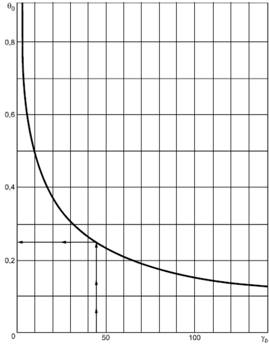
Рисунок М.1 - График для определения \theta_0
