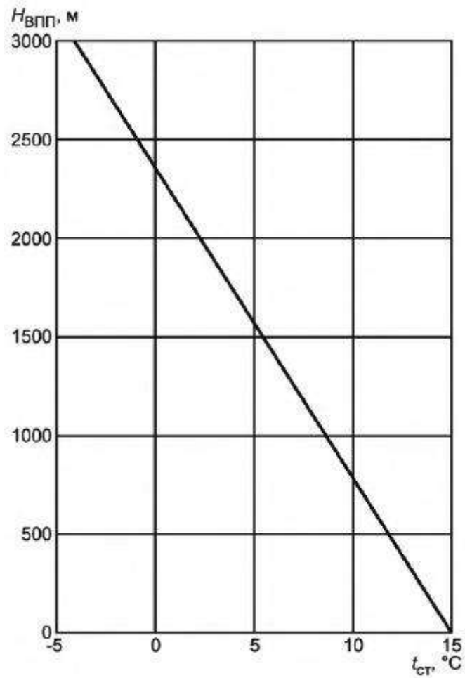
Рисунок 4.1 - Зависимость температуры стандартной атмосферы от высоты аэродрома над уровнем моря
