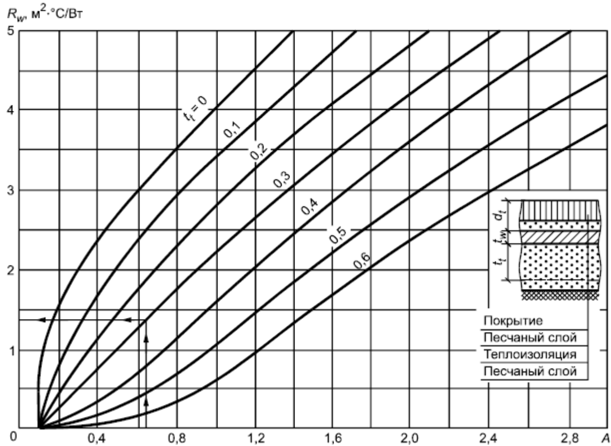
Рисунок Д.2 - Номограмма для определения термического сопротивления теплоизоляции Приложение Е
