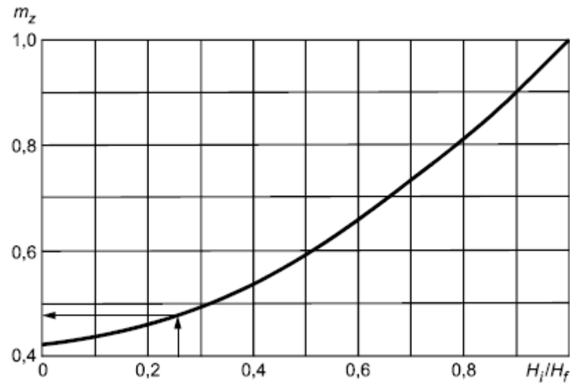
Рисунок Е.2 - График для определения коэффициента m_z
