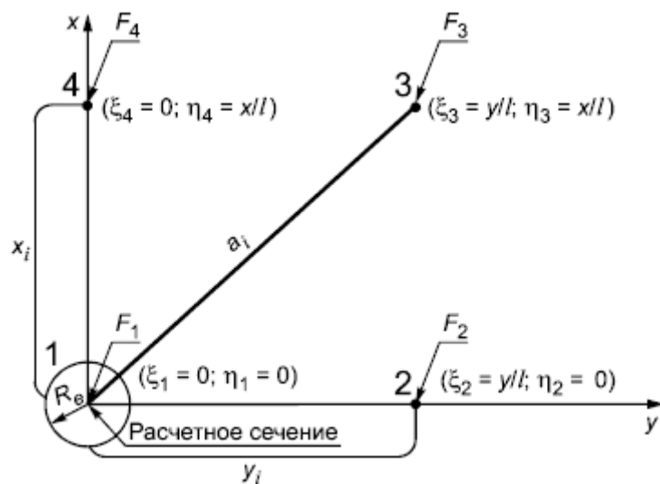
Рисунок 7.2 - Расчетная схема параметров нагружения опор ВС - для сечений железобетонных плит с ненапрягаемой арматурой
