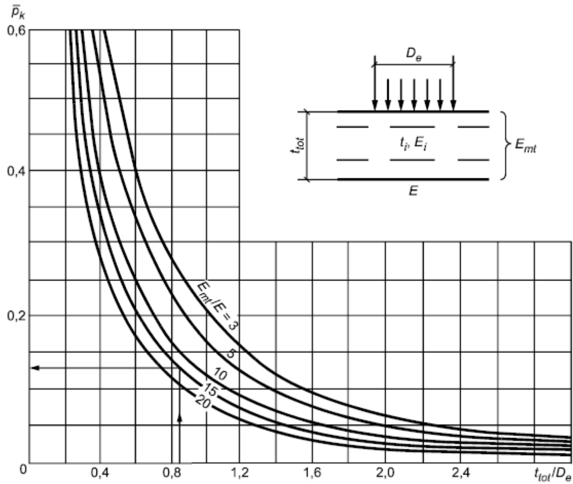
Рисунок Ж.1 - Номограмма для определения удельных контактных давлений \bar{p}_k на поверхности грунтового основания нежестких покрытий Ж.6 Эквивалентное расстояние a_e , м, следует определять по формуле
