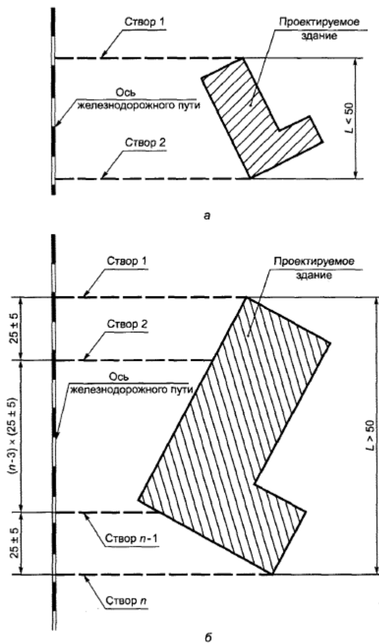
Рисунок Б.1 - Створы измерения вибрации при длине здания до 50 м (а) и свыше 50 м (б)
