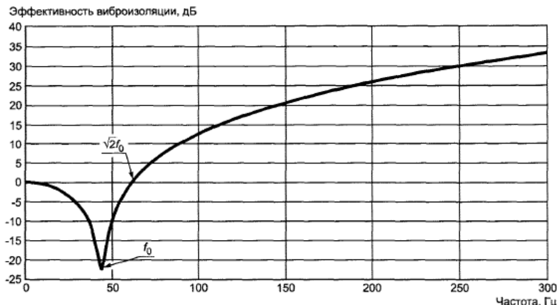
Рисунок 7.1 - Эффективность одномассовой виброзащитной системы
