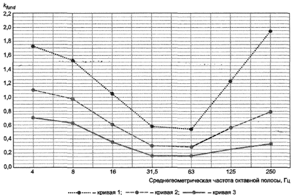
Рисунок 5.1 - Передаточная функция k_{fund}
