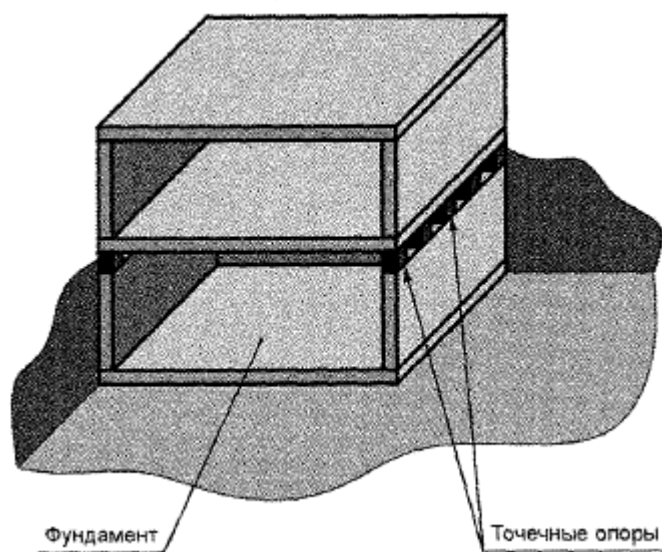
Рисунок 8.1 - Схема виброизоляции N 1
